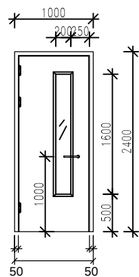
钢制复合单开门 (带视窗玻璃)
