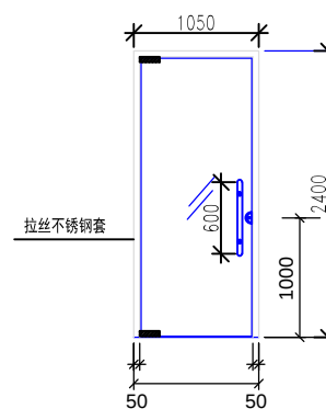
钢化玻璃单开门
