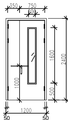
钢制复合子母门 (带视窗玻璃)
