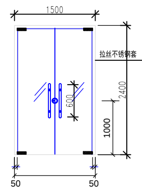
钢化玻璃双开门
