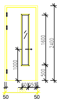
木制单开门 (带视窗玻璃)
