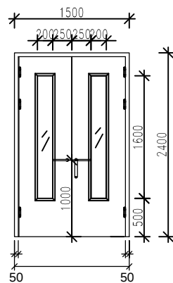
钢制复合双开门 (带视窗玻璃)
