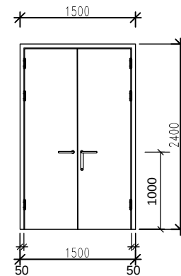
钢制复合双开门
