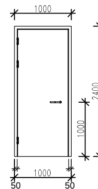
钢制复合单开门
