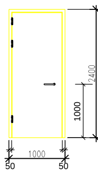
木制单开门
