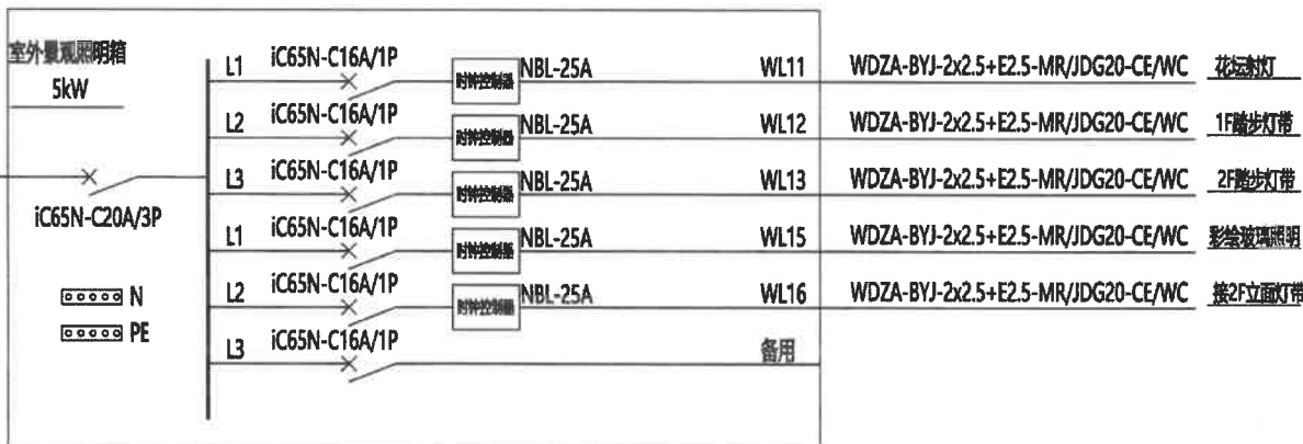
室外景观照明箱系统图 室外景观照明箱
