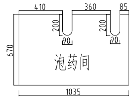
泡药间 样图一 格栅花纹盖板厚度44 mm
