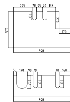
污泥间 样图六 格栅花纹盖板厚度44 mm
