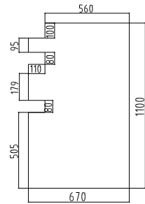
污泥间 样图四 格栅花纹盖板厚度90 mm
