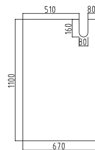
污泥间 样图五 格栅花纹盖板厚度90 mm
