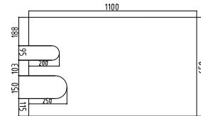
污泥间 样图七 格栅花纹盖板厚度44 mm
