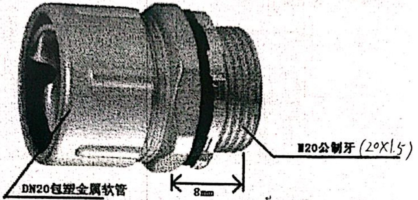
A图 入盒接头
