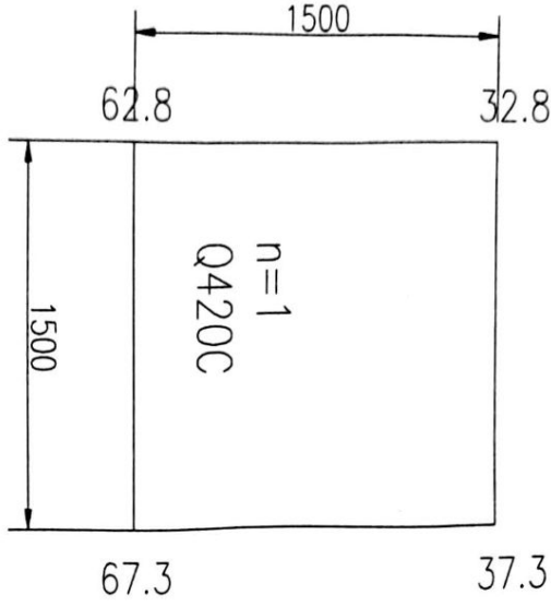
ZK53(左) 支座垫板 t72*1500*1500
