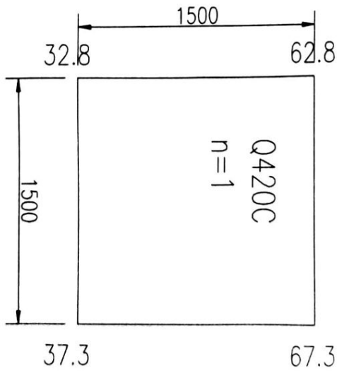
桥墩QC0 支座垫板 t75*1500*1500
