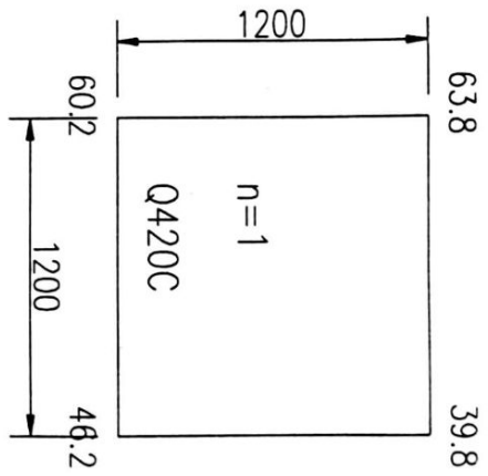
ZK51 (右) 支座垫板 t72*1200*1200
