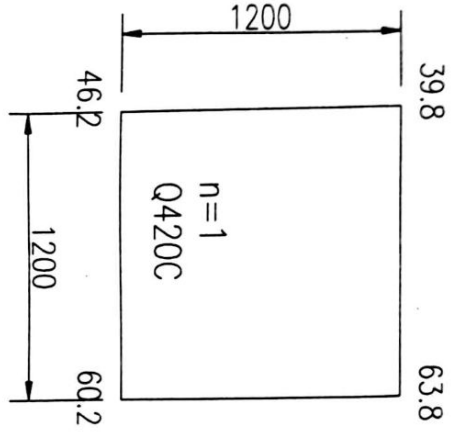
ZK51 (左) 支座垫板 t72*1200*1200
