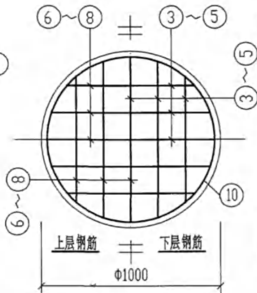
底板平面配筋图
