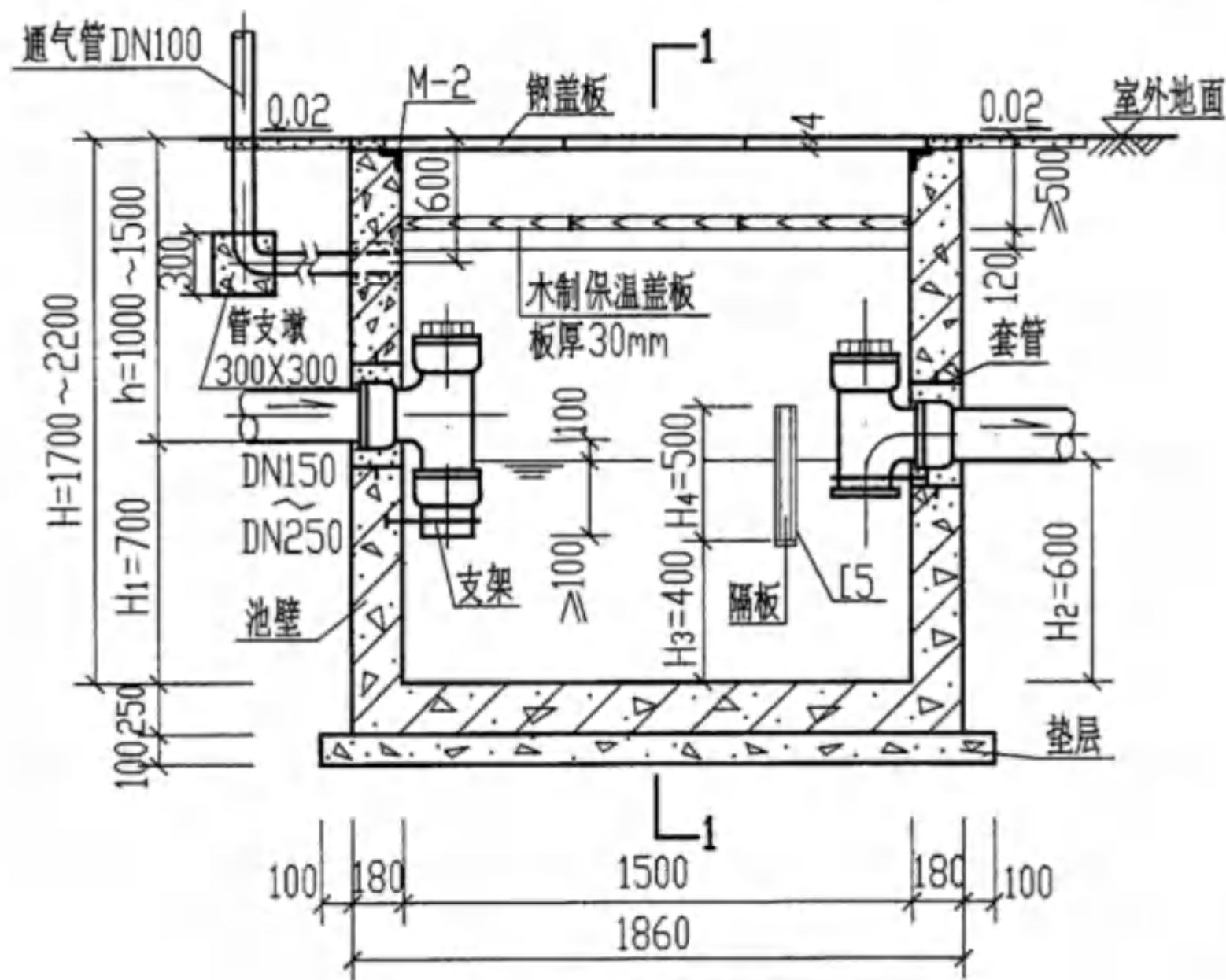
GG-1F, 1SF 保温做法
