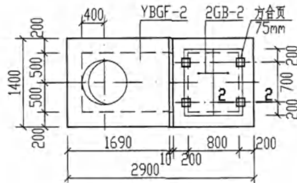
GG-3F. 3SF 盖板平面布置图
