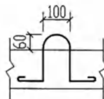
吊钩大样图
