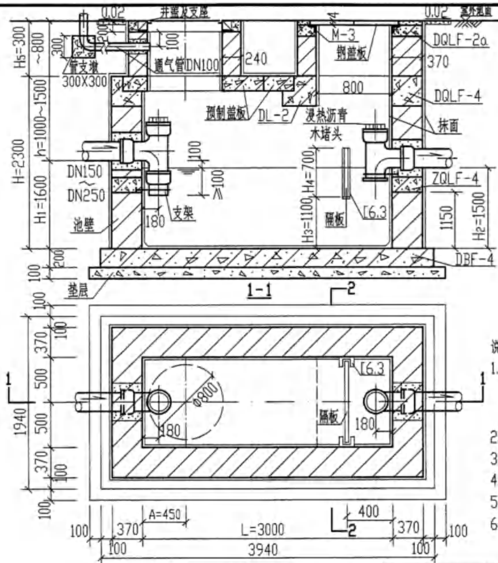
ZG-4F 平面图
