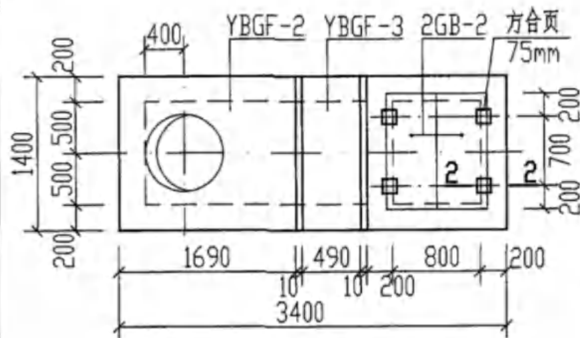
GG-4F. 4SF 盖板平面布置图
