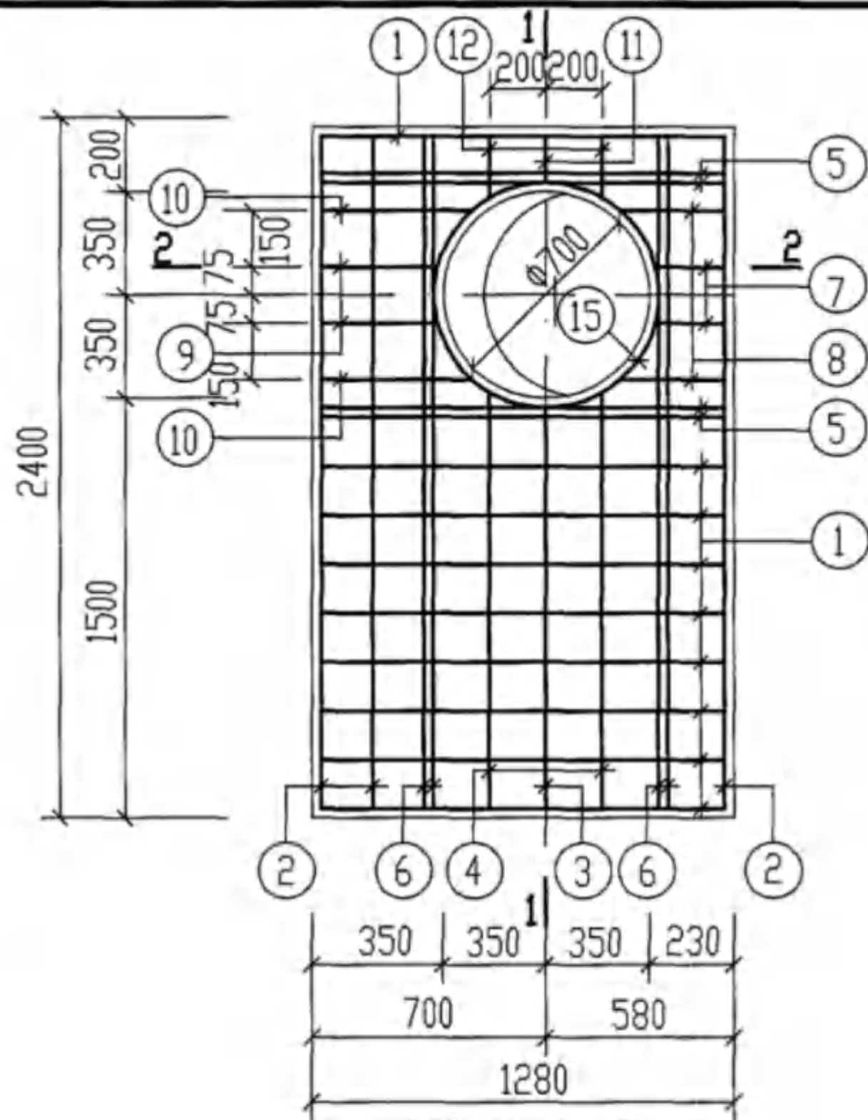
DGB-3a. 6a. 7a
