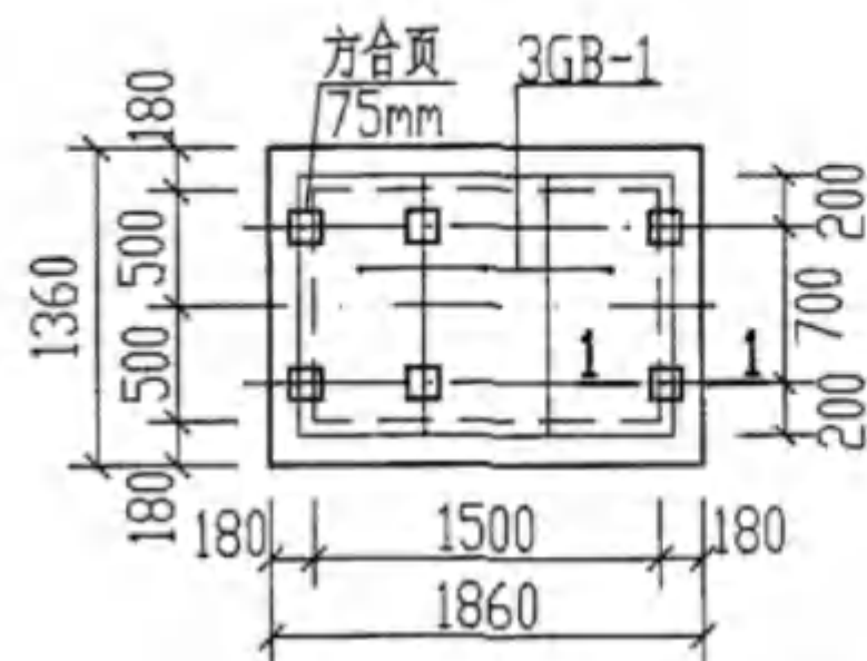
GG-1F. 1SF 盖板平面布置图
