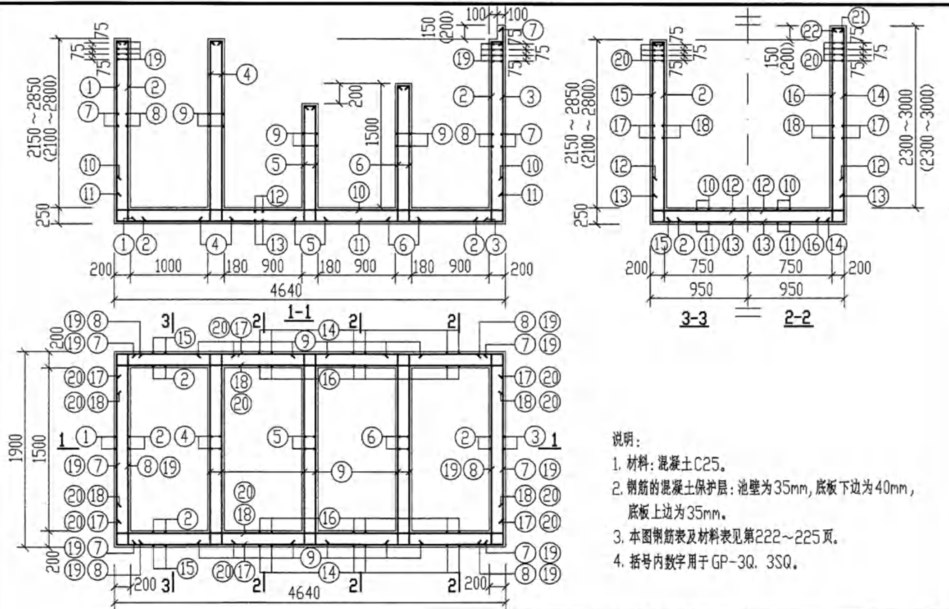
GP-3, 3S, 3Q, 3SQ平面配筋图
