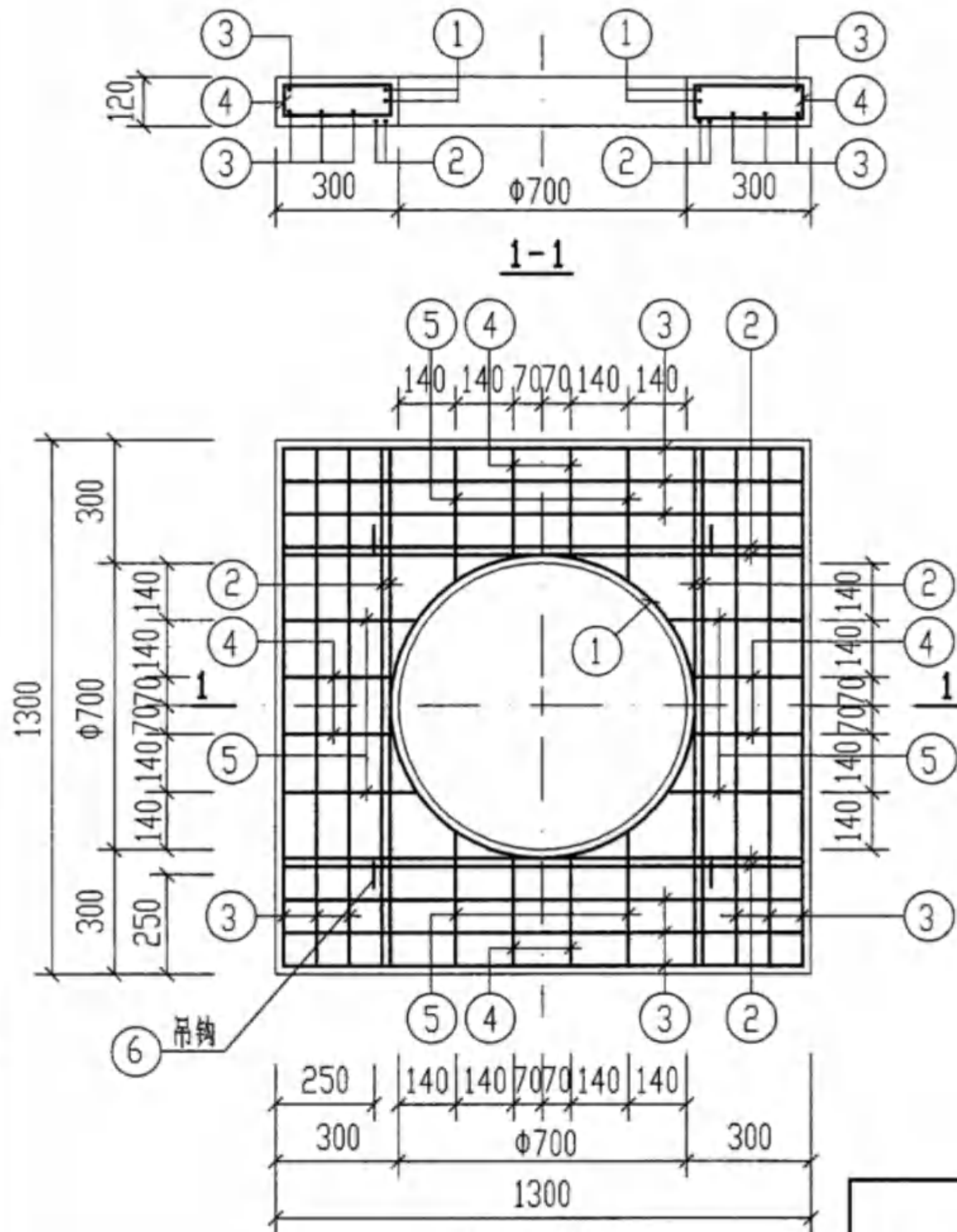
井圈(七)配筋图
