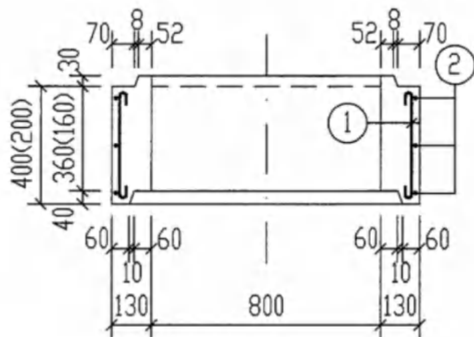
1-1 用于JQ-1 (JQ-2)
