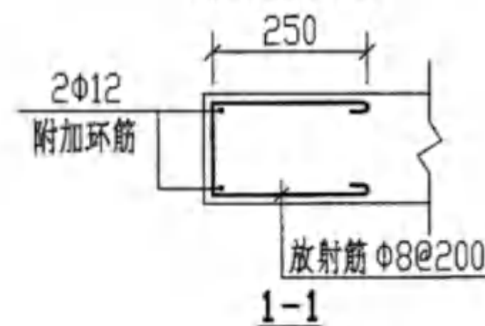
300 ≤ d 3 ≤ 1000 洞口加强大样图 (钢筋混凝土池壁)
