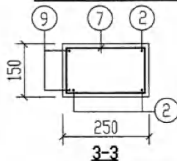
YBG-5. YBGF-5 配筋图(无覆土和有覆土)
