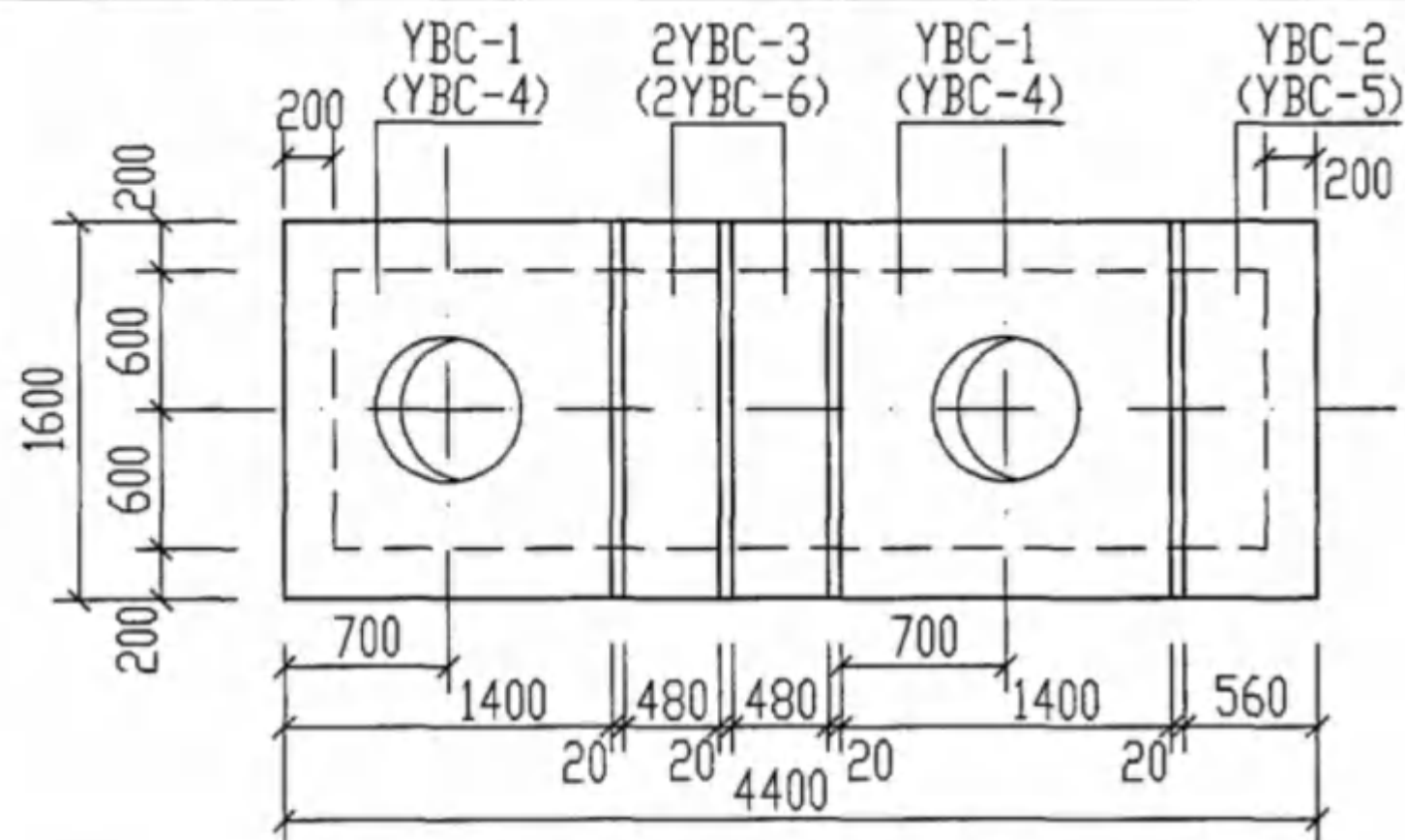
GC-2, 2S (GC-2Q, 2SQ) 盖板平面布置图
