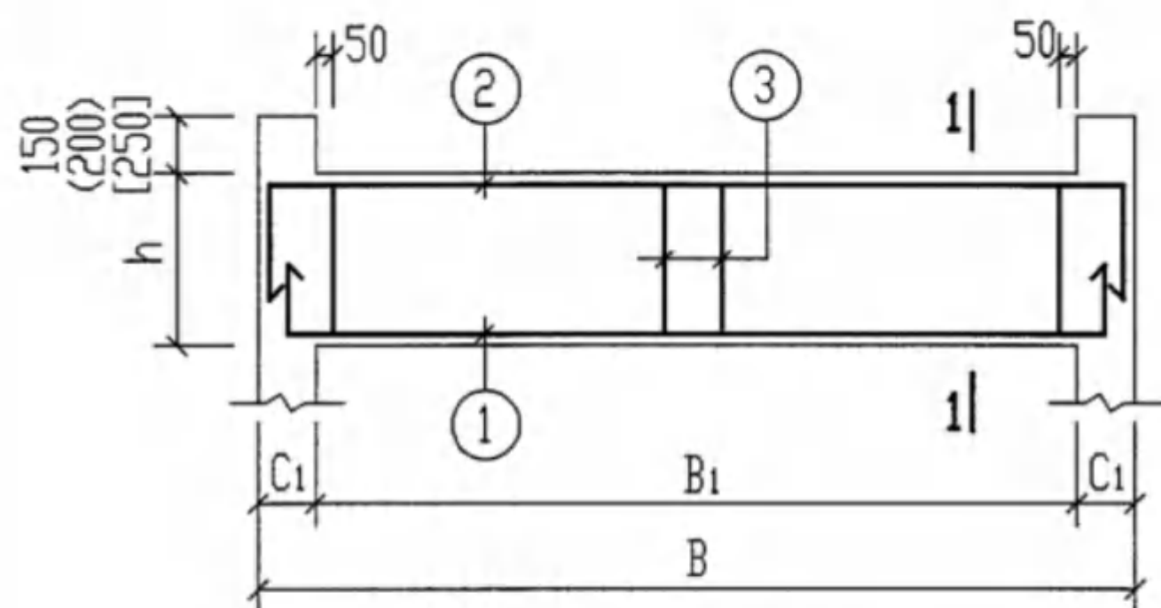
现浇梁XL-1~XL-6配筋图
