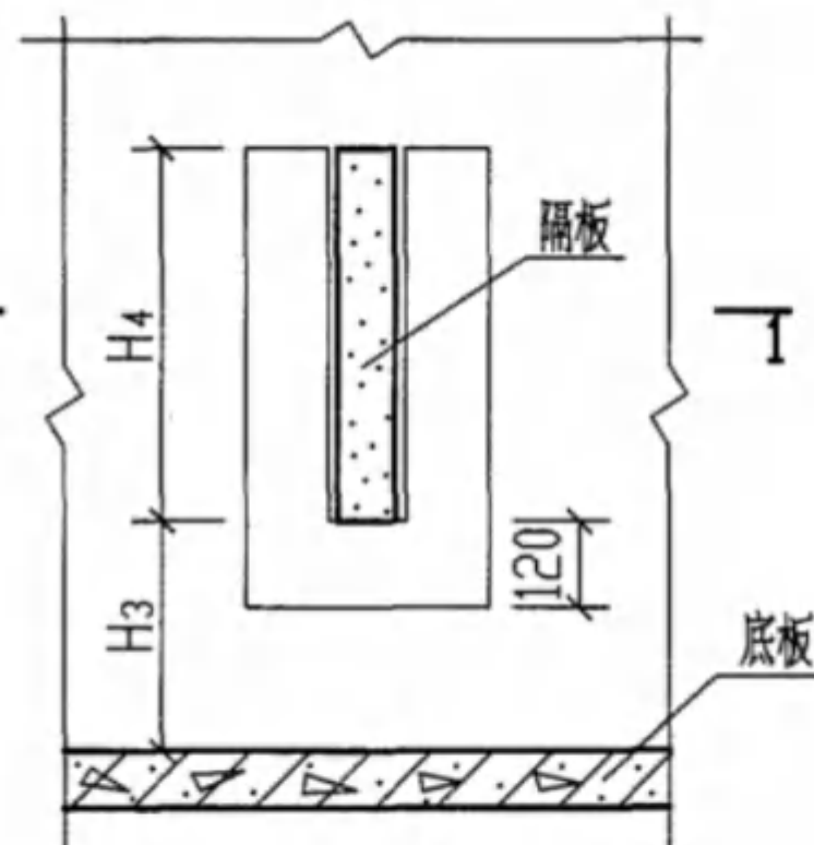
砖池壁固定隔板大样图 B
