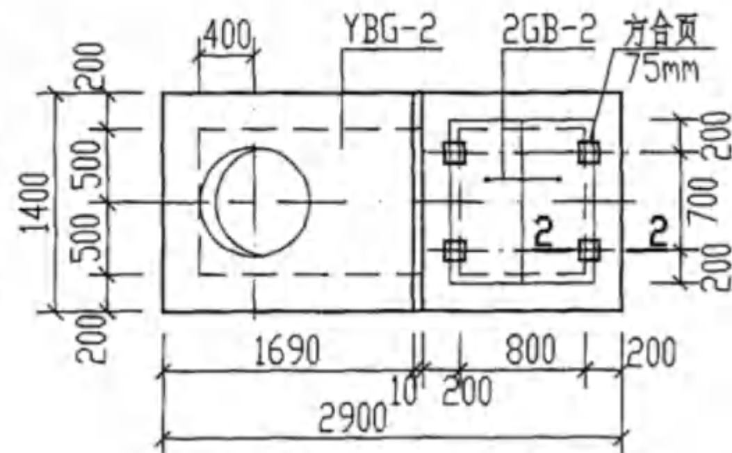
GG-3. 3S 盖板平面布置图
