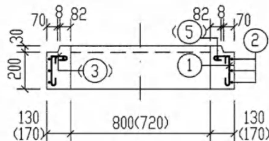
1-1 用于JQ-4 (JQ-5)
