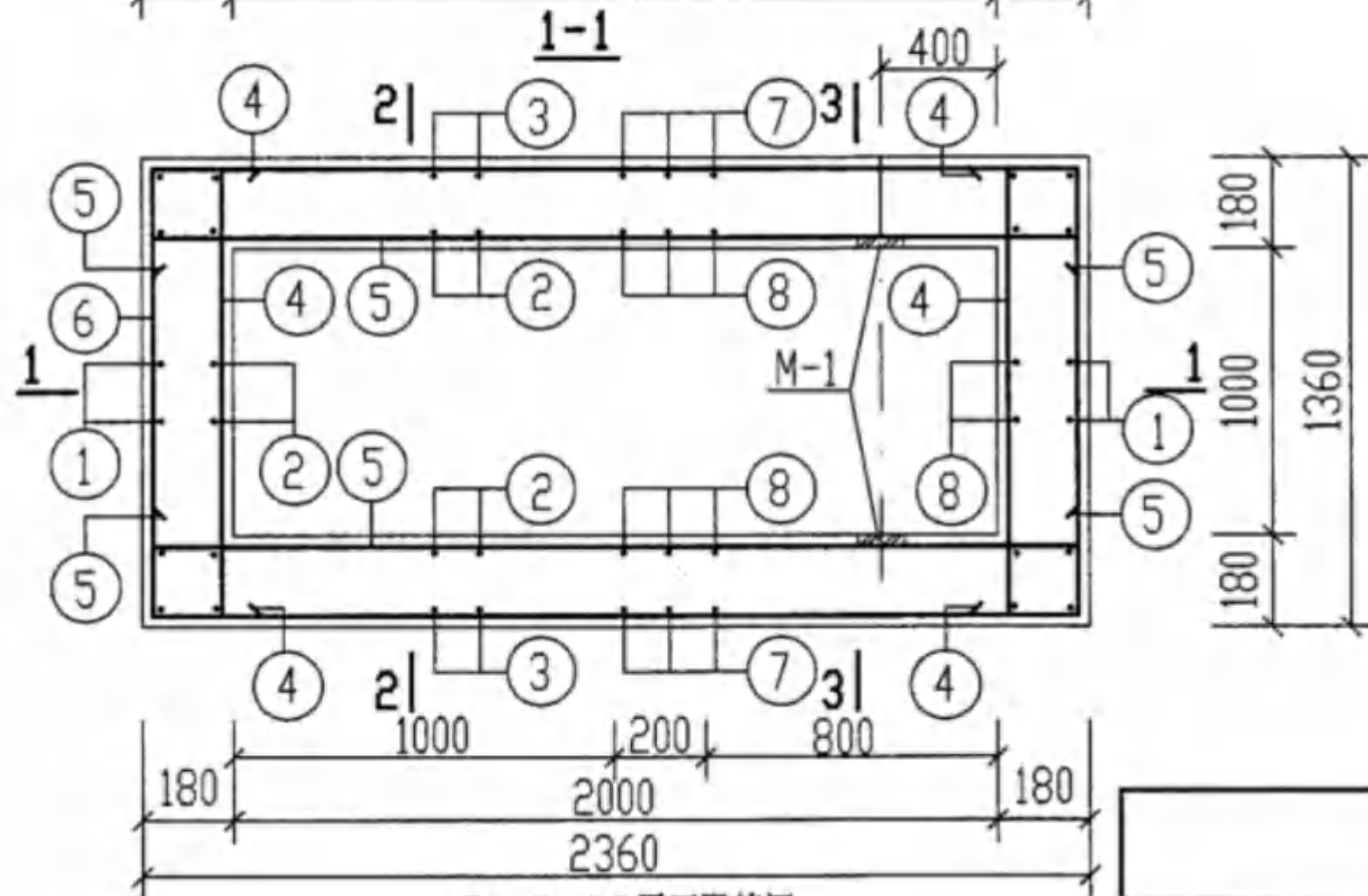
GG-2, 2S 平面配筋图
