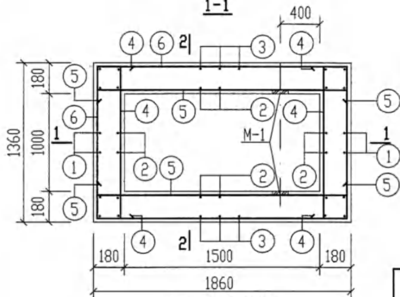
GG-1. 1S 平面配筋图
