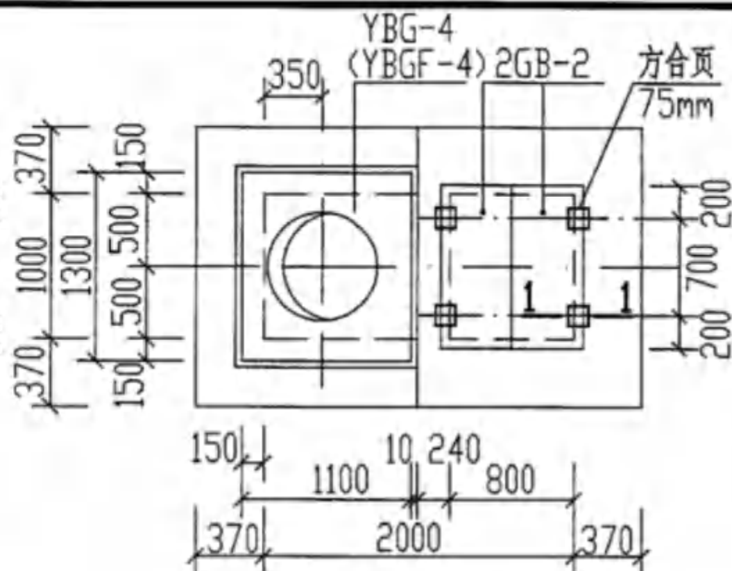
ZG-2. (ZG-2F) 盖板平面布置图
