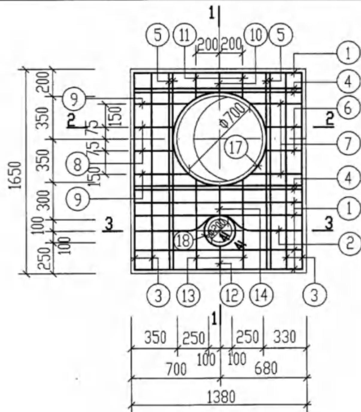
DGB-1. 4 下层钢筋
