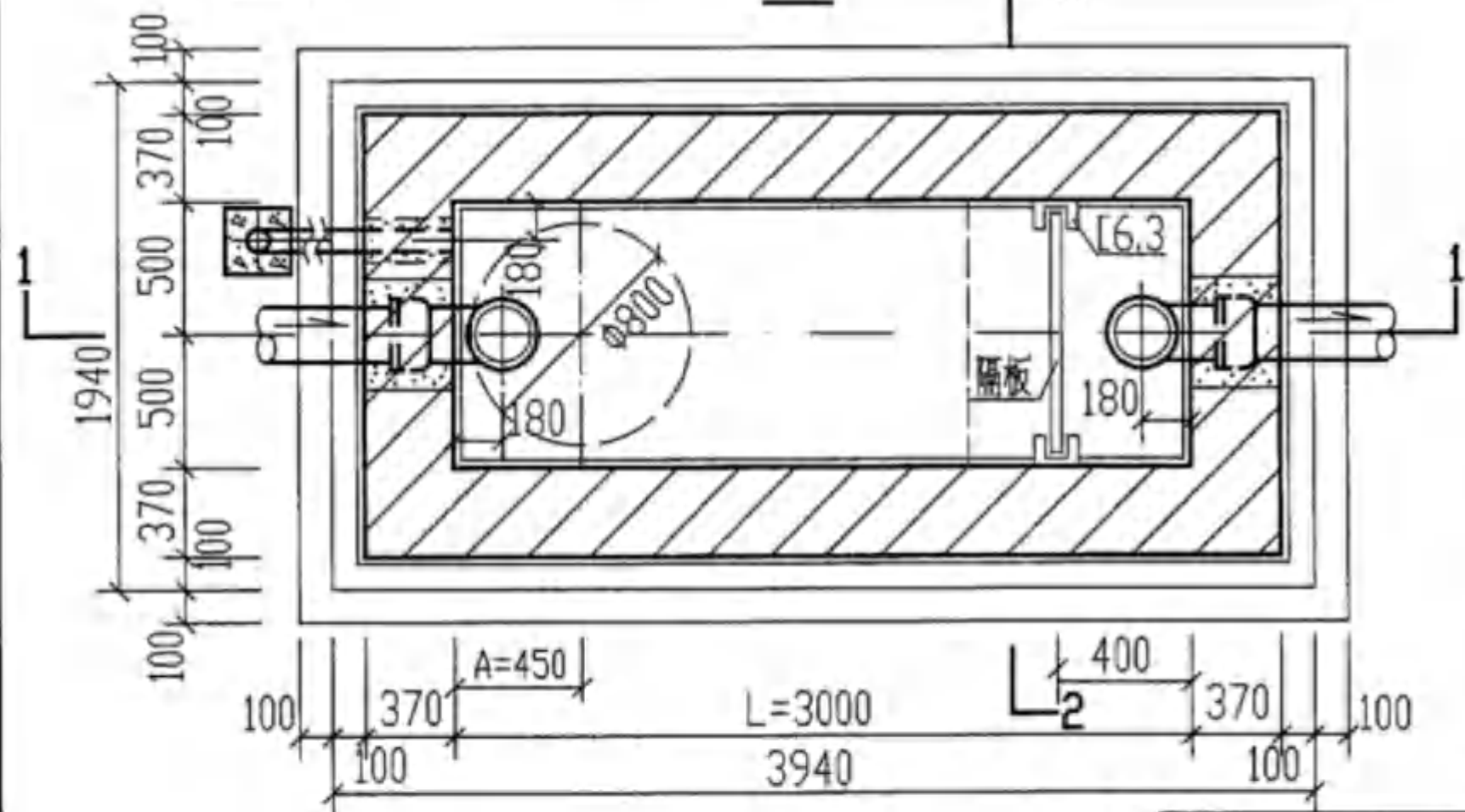
ZG-4 平面图
