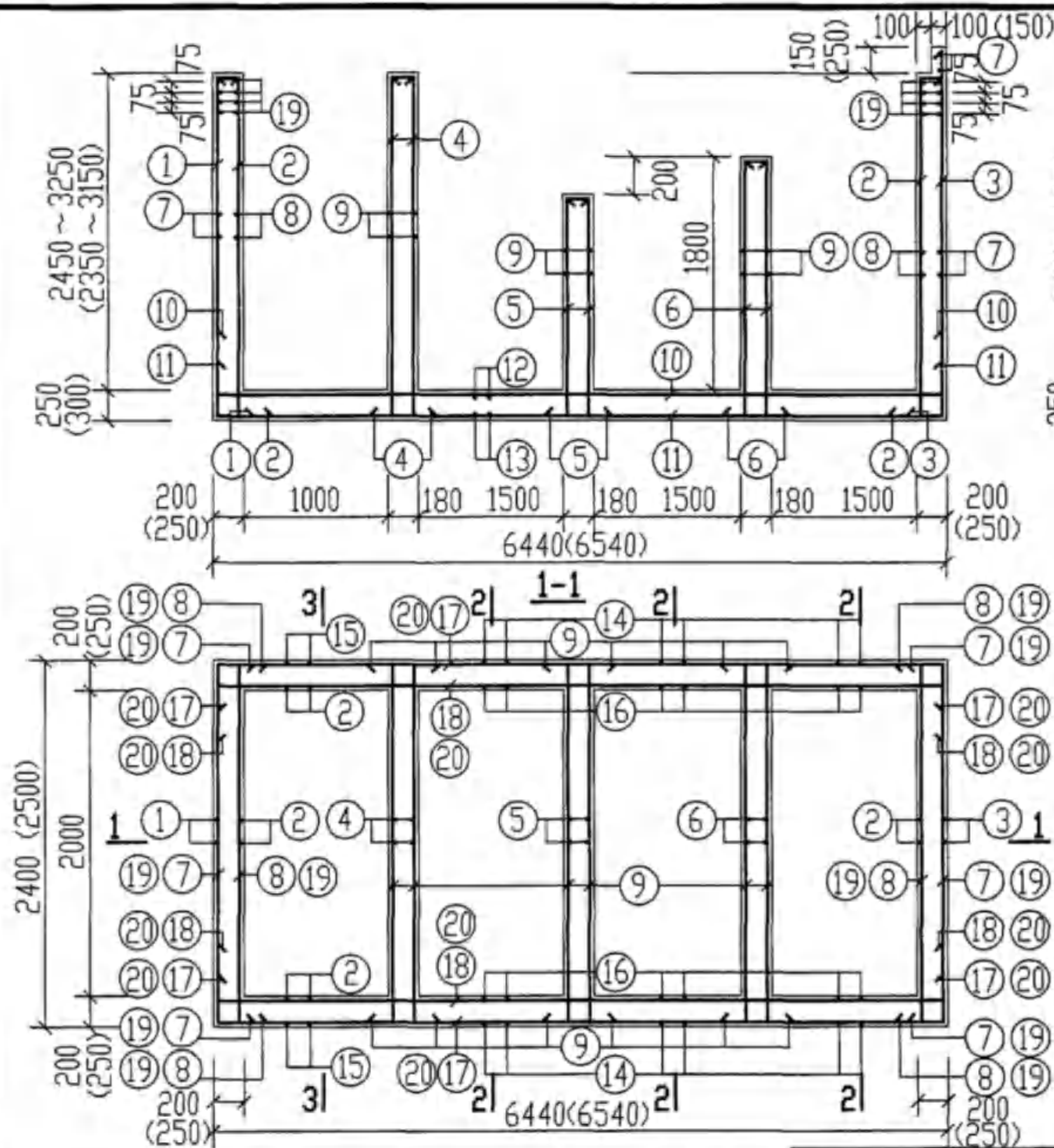
GP-6, 6S, 6Q, 6SQ 平面配筋图
