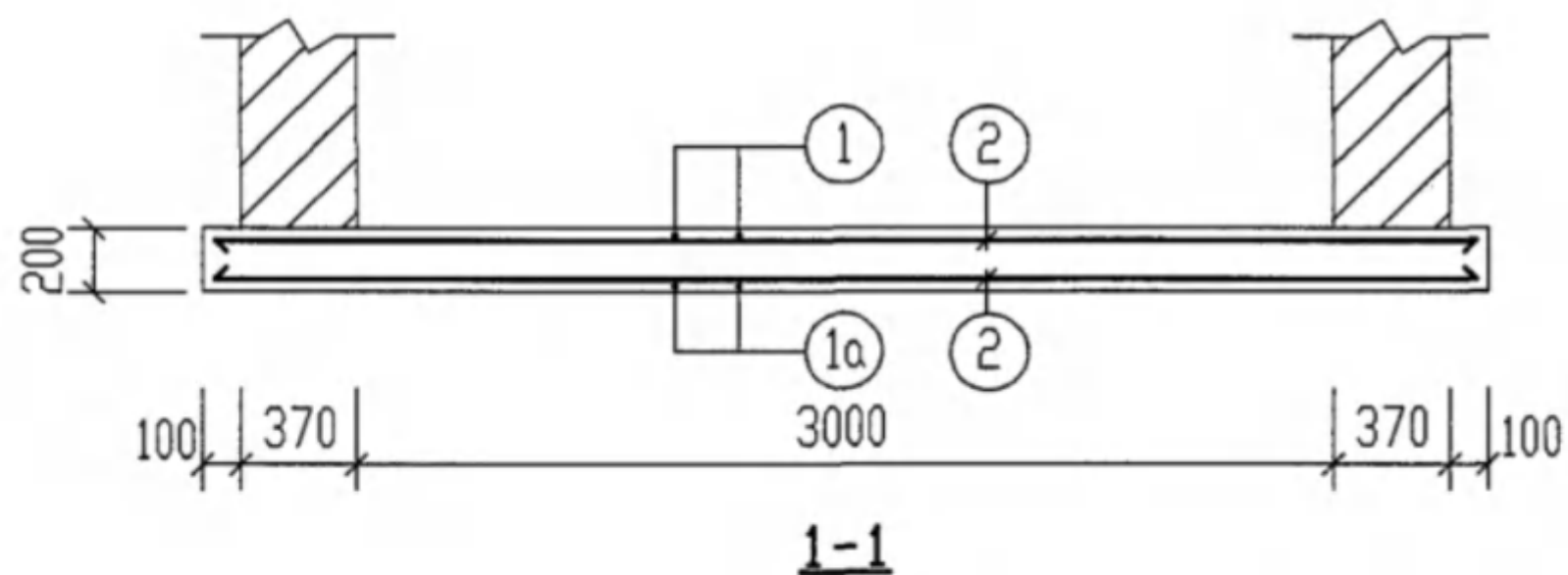
底板 DB-1 配筋图
