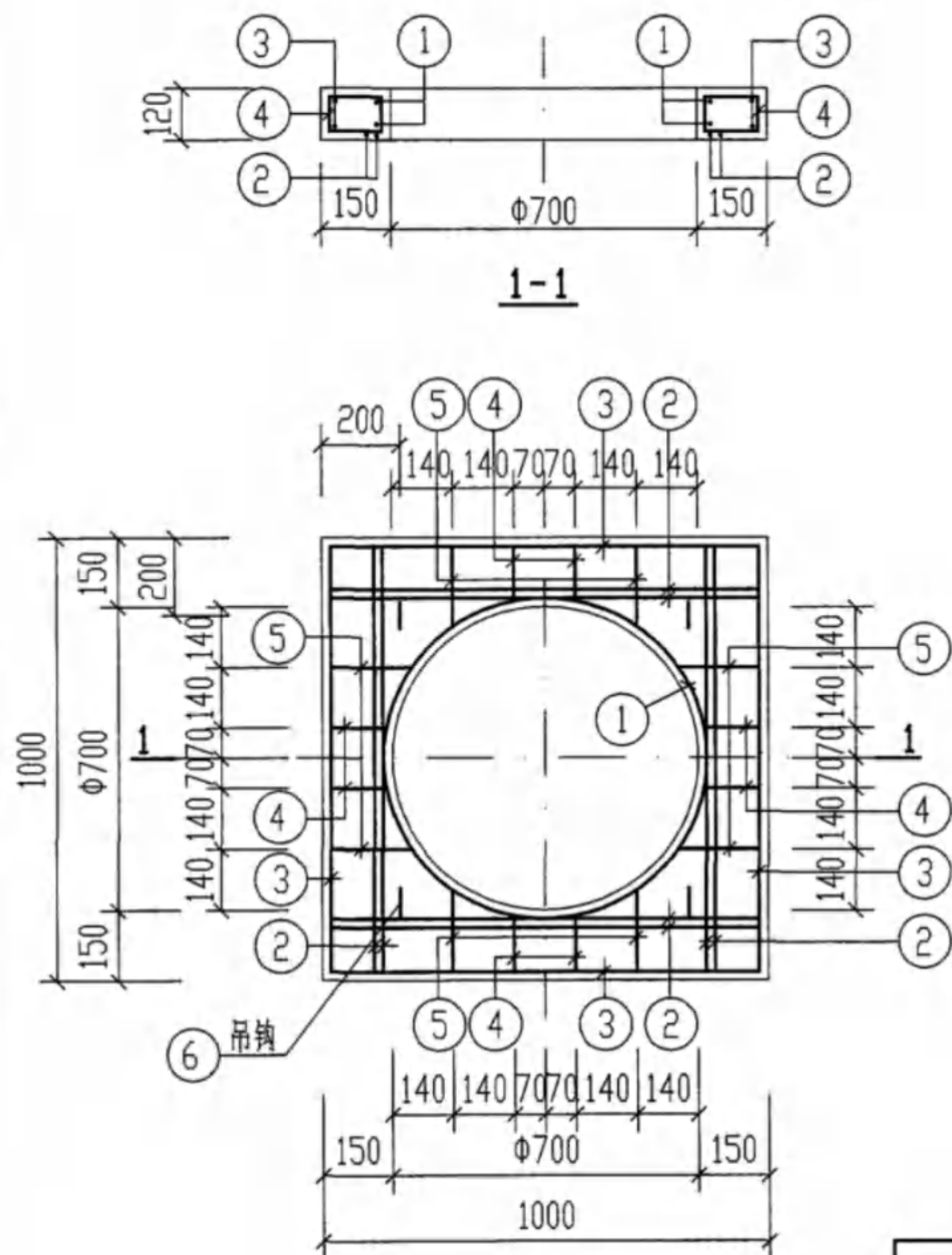
井圈(六)配筋图
