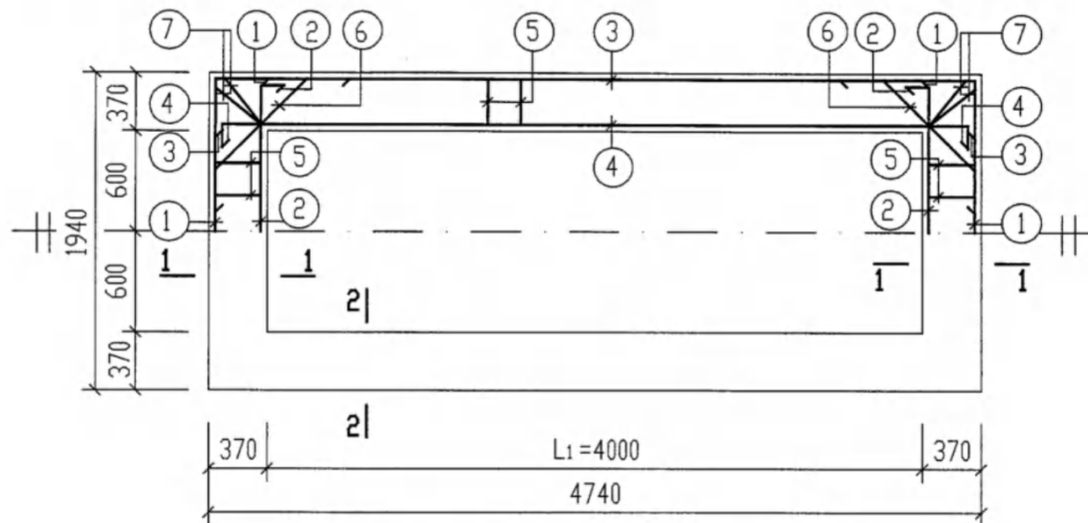
中圈梁 ZQL-2. 2a ZQLF-2. 2a 配筋图
