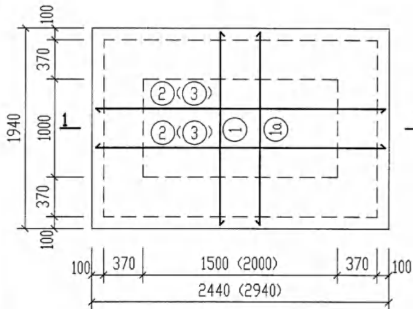
底板DB-1 (DB-2)配筋图
