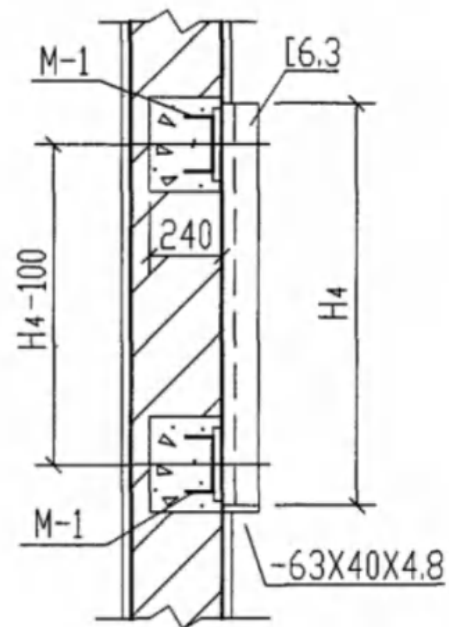
中间隔板预埋件大样图 A
