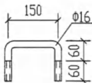
把手大样图
