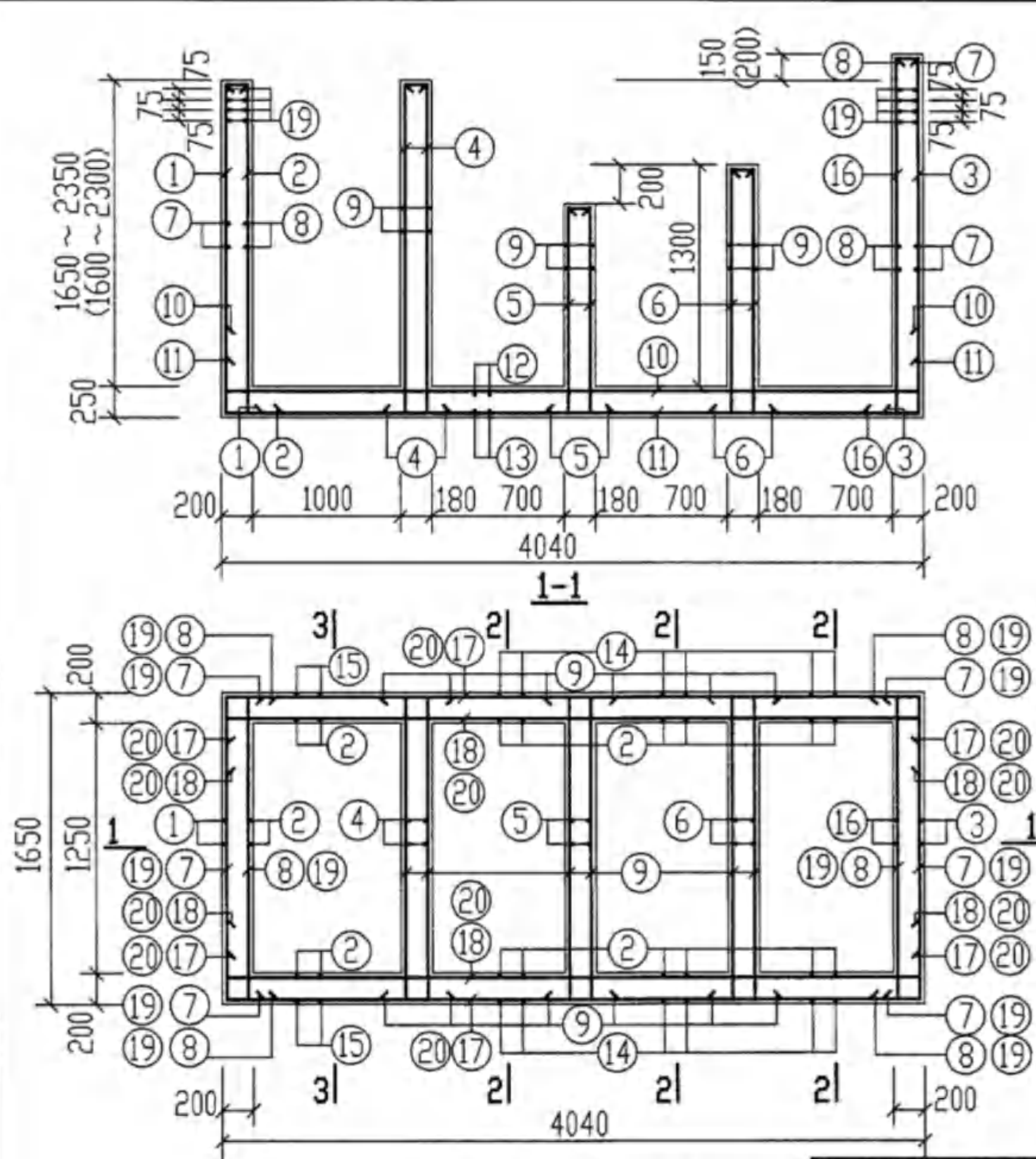
GP-2, 2S, 2Q, 2SQ 平面配筋图
