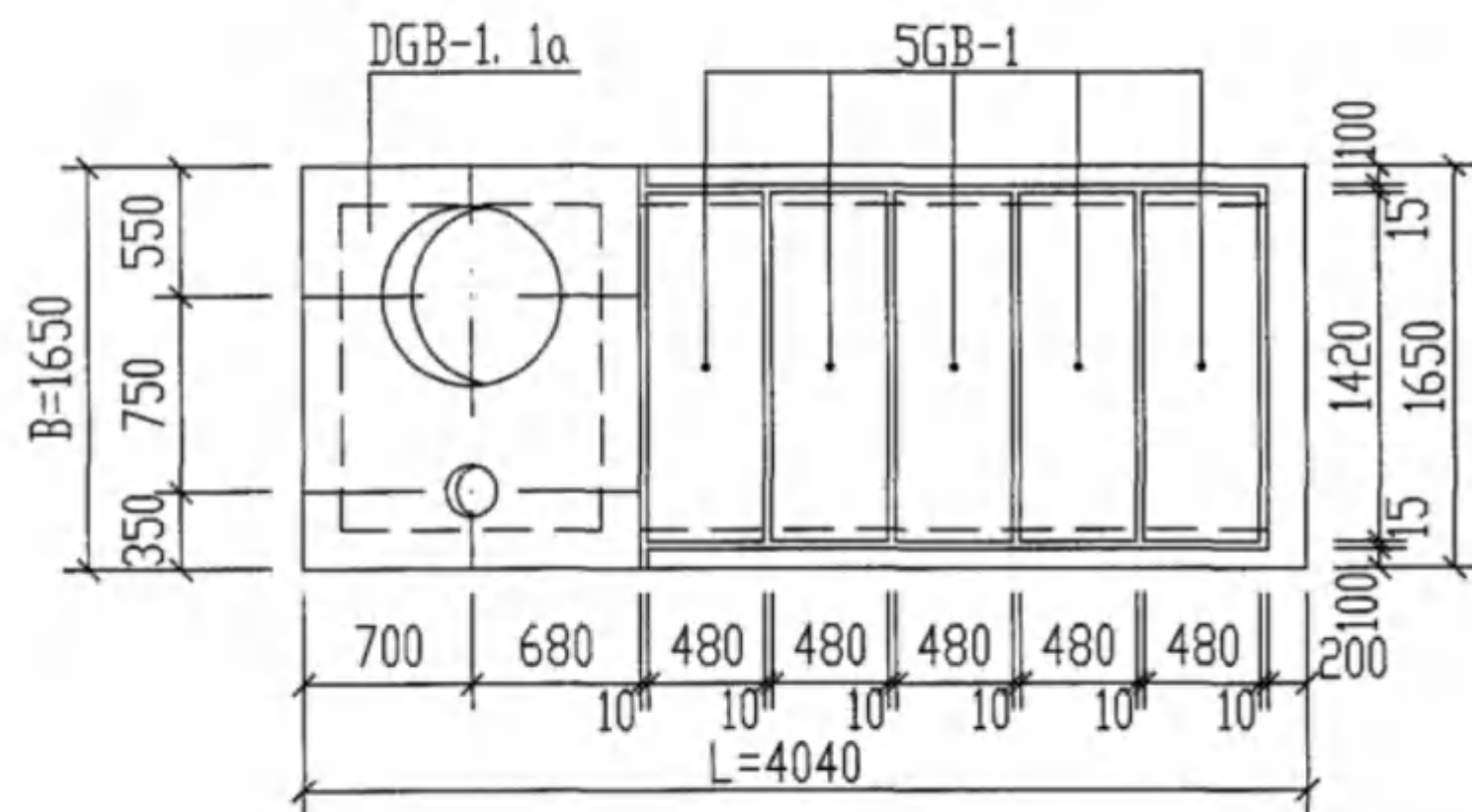
GP-1. 1S GP-2. 2S池盖板平面布置图
