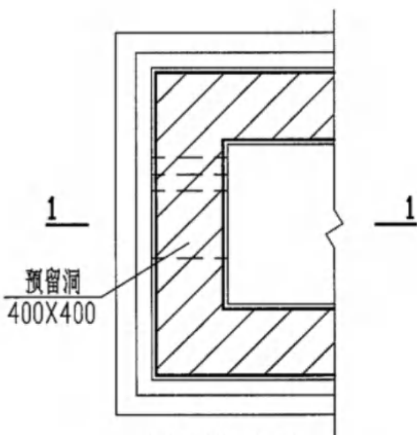
隔油池局部平面图
