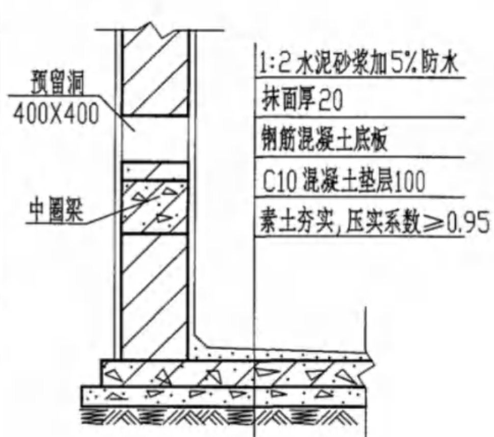
池底做法 (用于无地下水)
