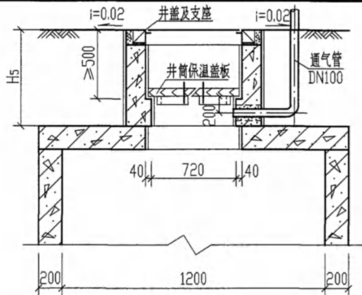
钢筋混凝土保温井口
