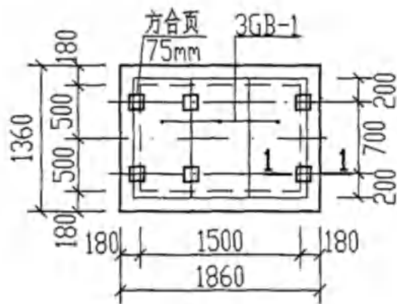
GG-1. 1S 盖板平面布置图
