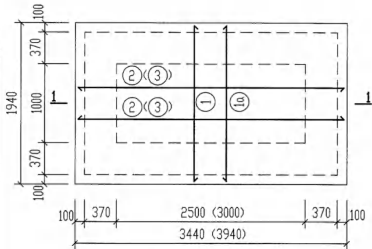
底板 DBF-3 (DBF-4) 配筋图
