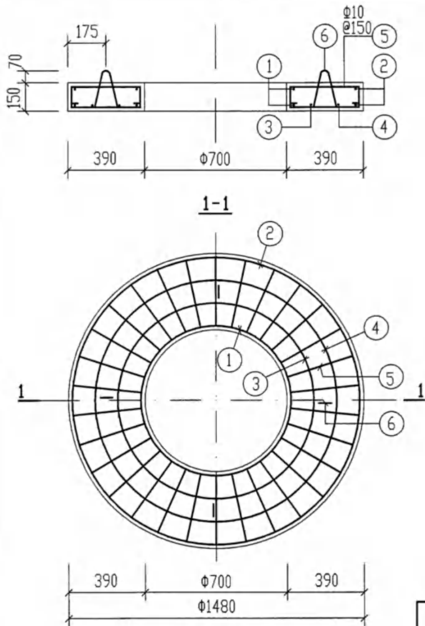
井圈(四)配筋图
