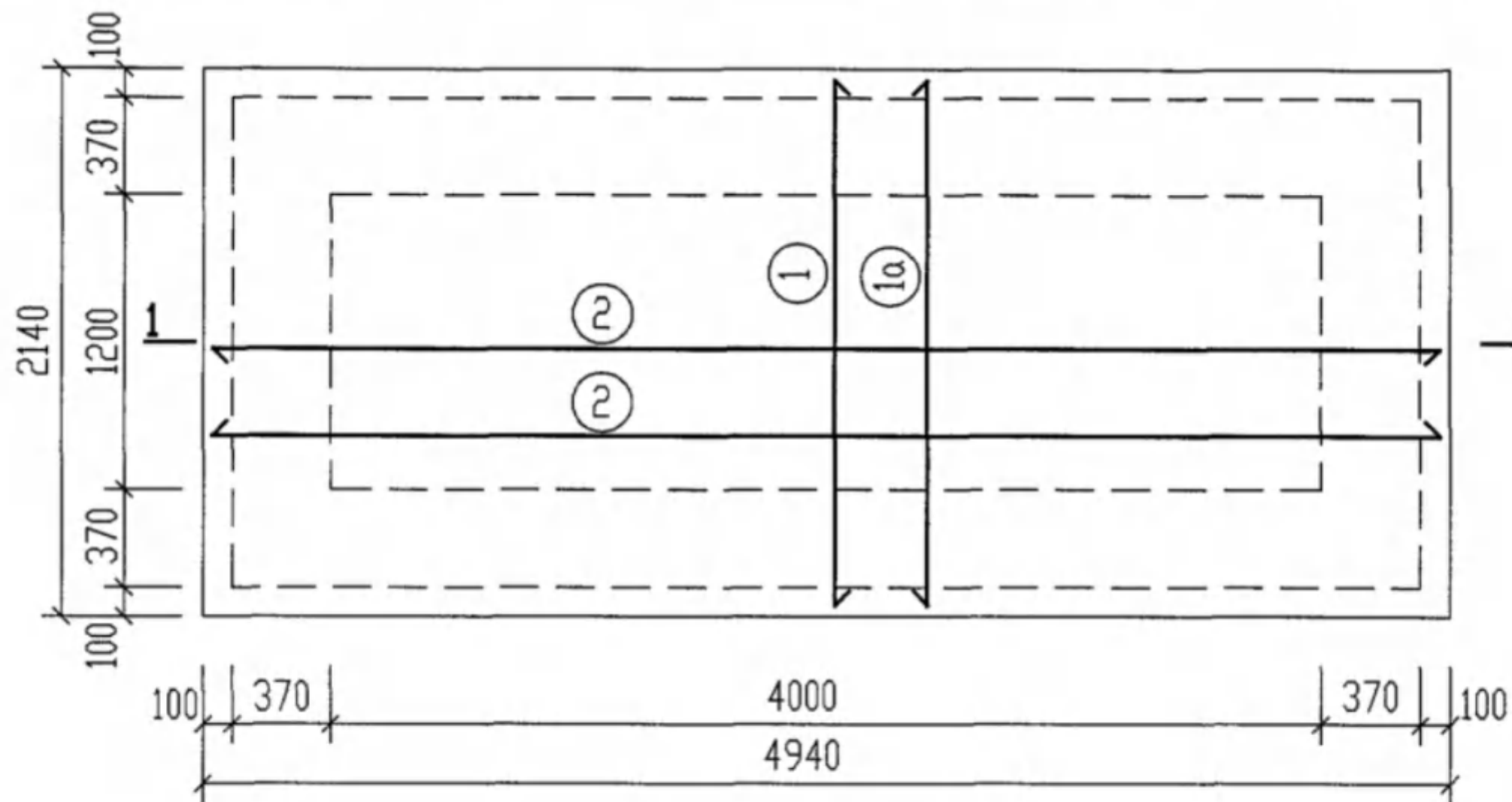
底板 DB-2 配筋图
