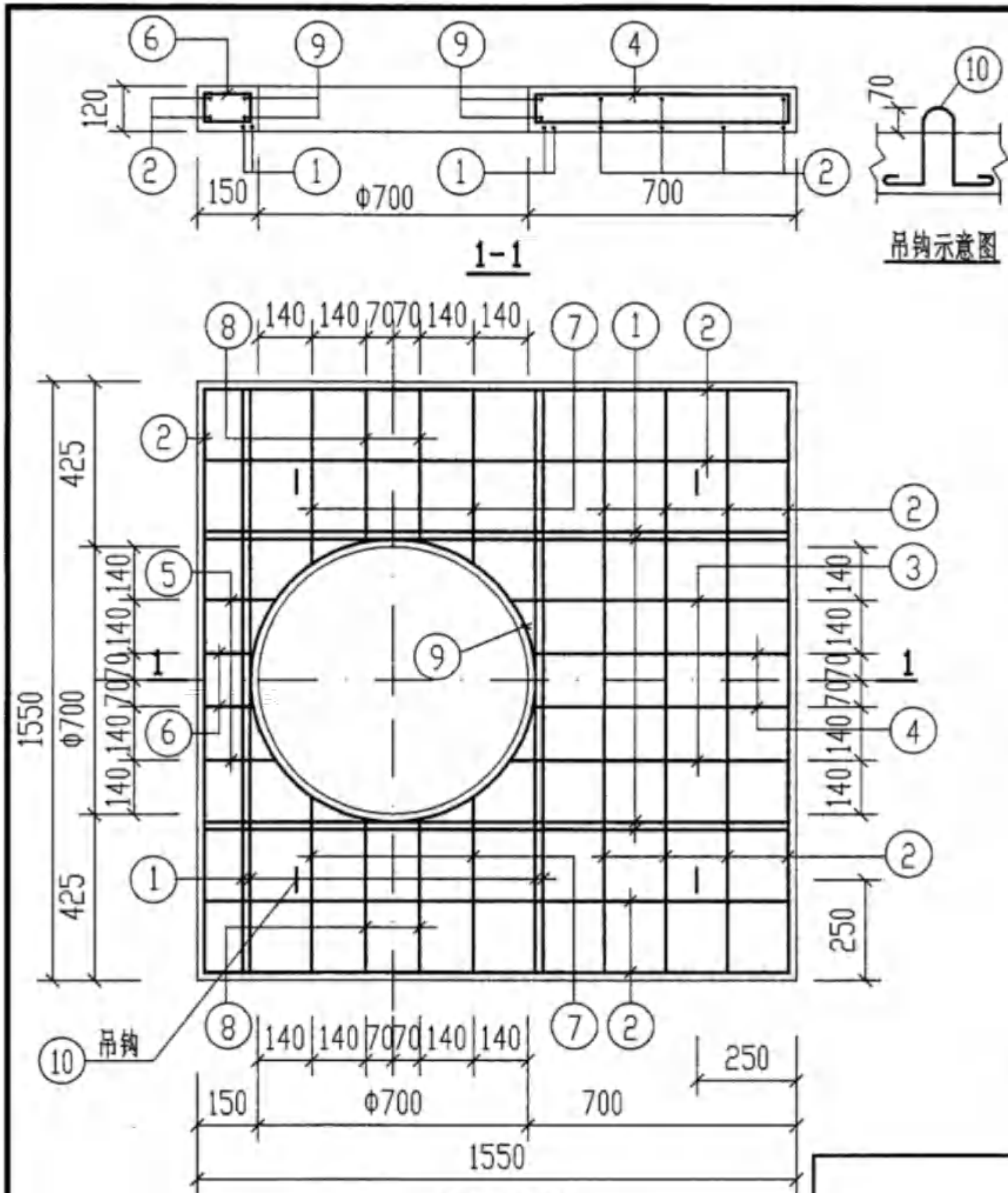
井圈(十)配筋图
