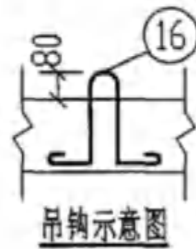
DGB-3a. 6a. 7a
