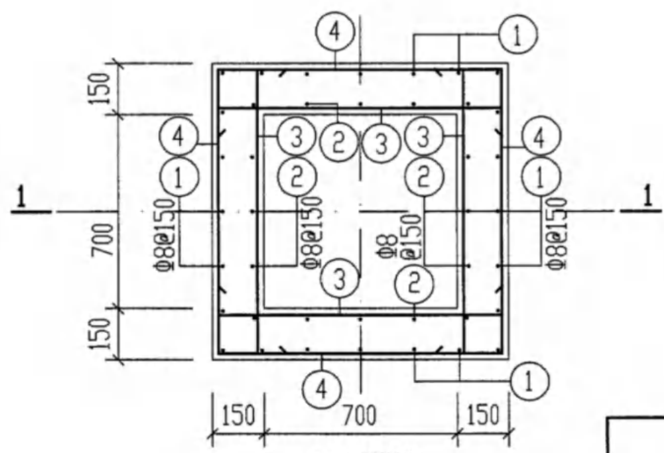
GF-1配筋图
