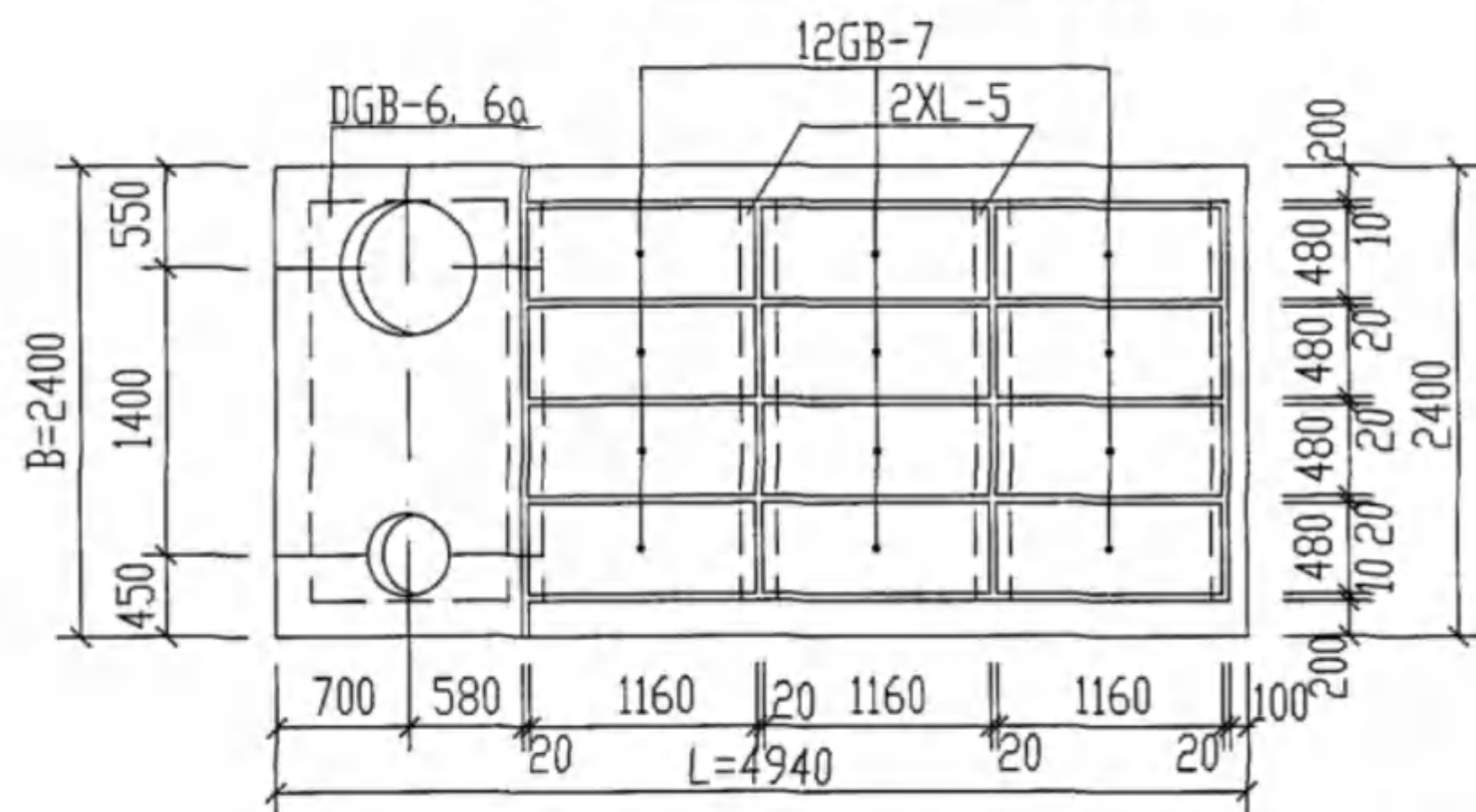
GP-4Q, 4SQ 池盖板平面布置图
