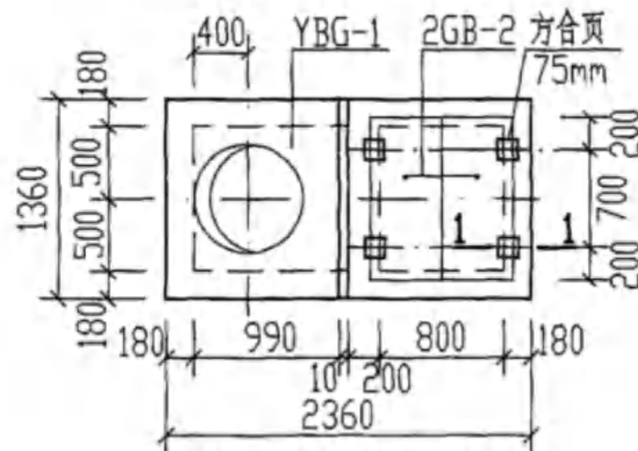
GG-2. 2S 盖板平面布置图
