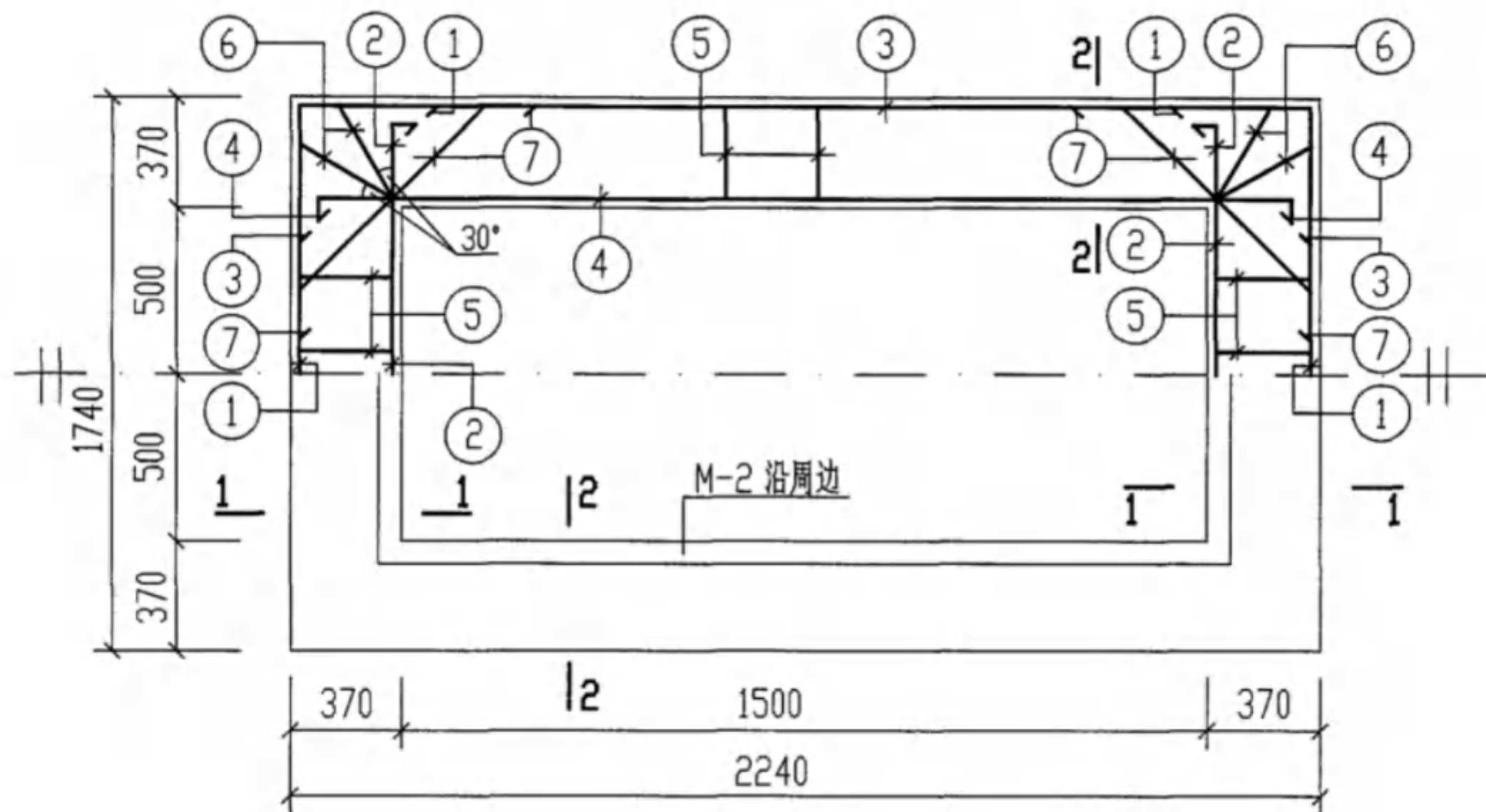
顶圈梁 DQL-1, DQLF-1 配筋图
