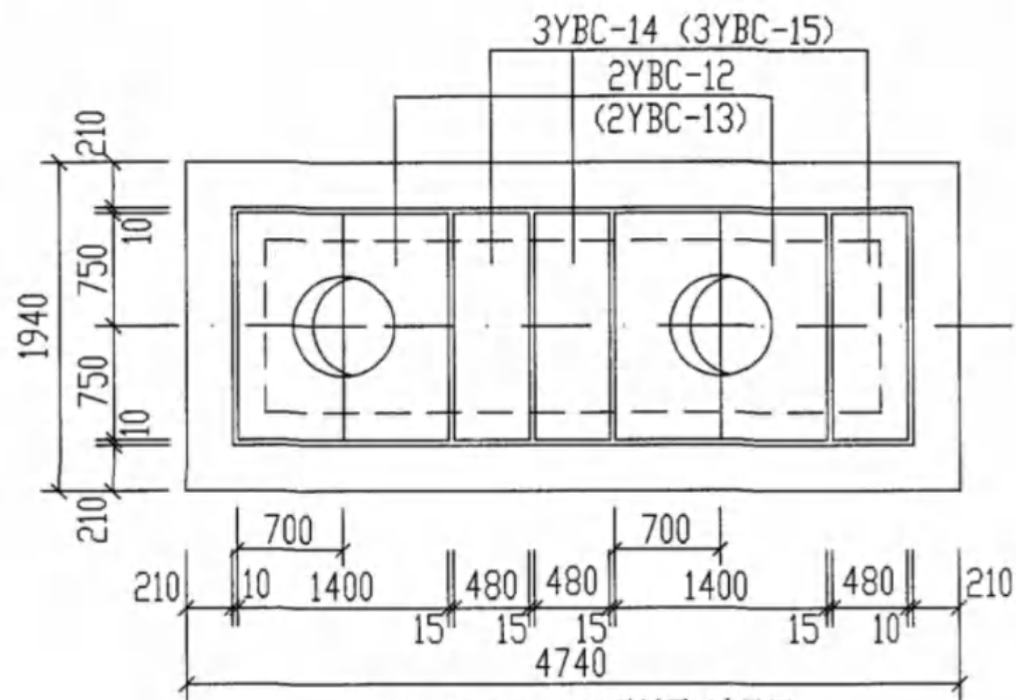
ZC-2. (ZC-2Q) 盖板平面布置图
