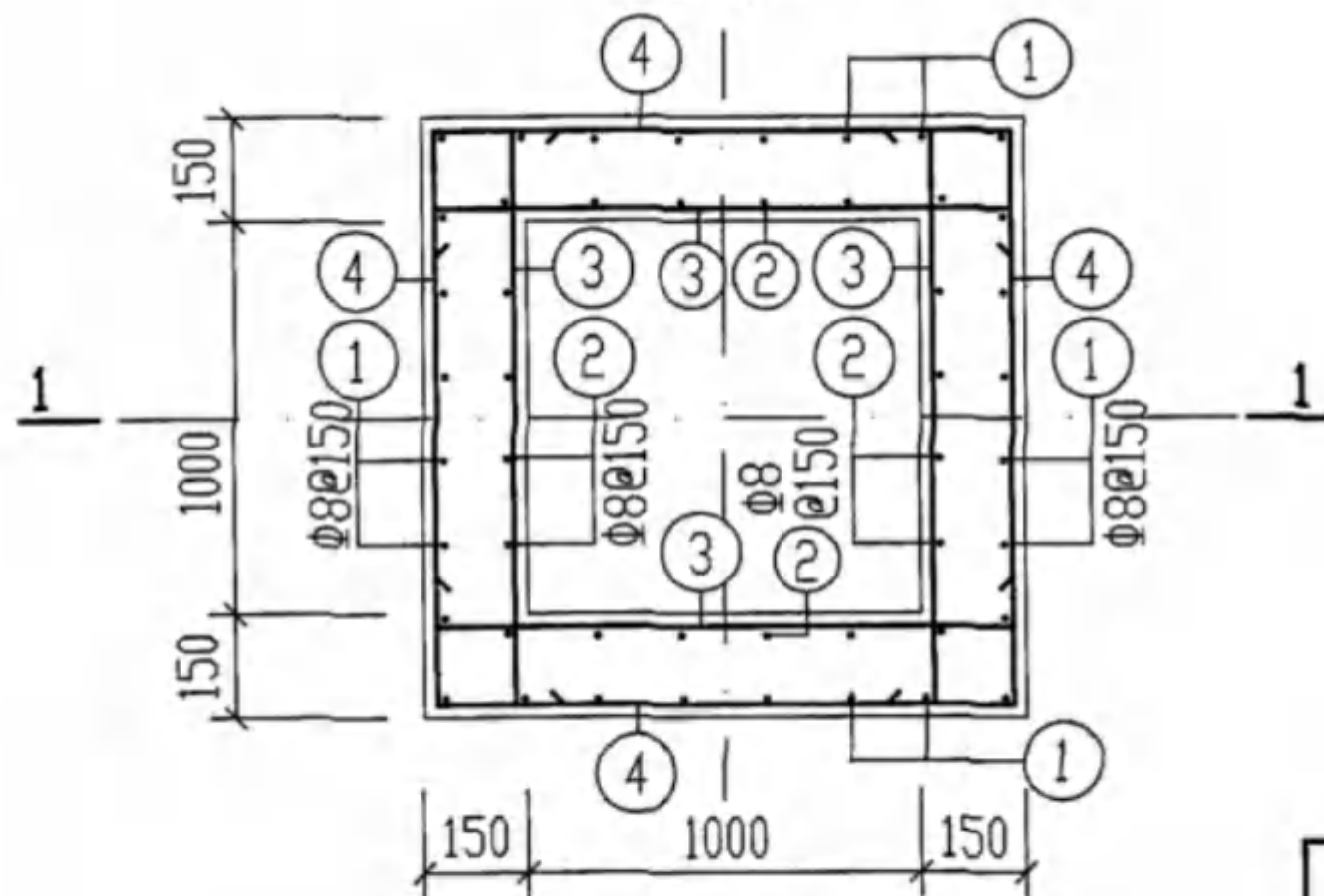
GF-2 配筋图
