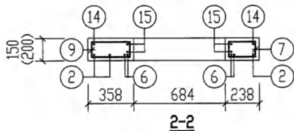
DGB-2a, 5a 下层钢筋
