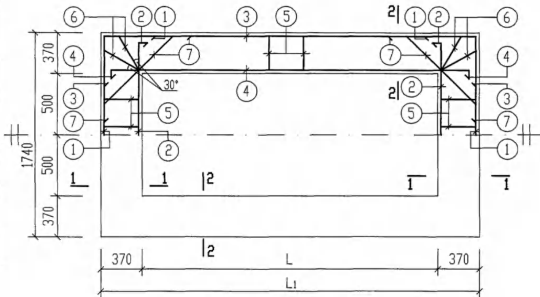
中圈梁 ZQL-1~4, ZQLF-1~4 配筋图
