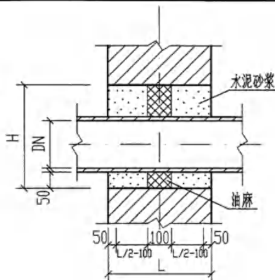
管道穿砖壁预留洞
