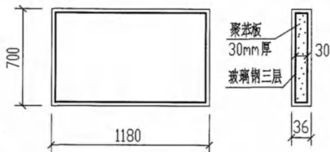
中间隔板大样图
