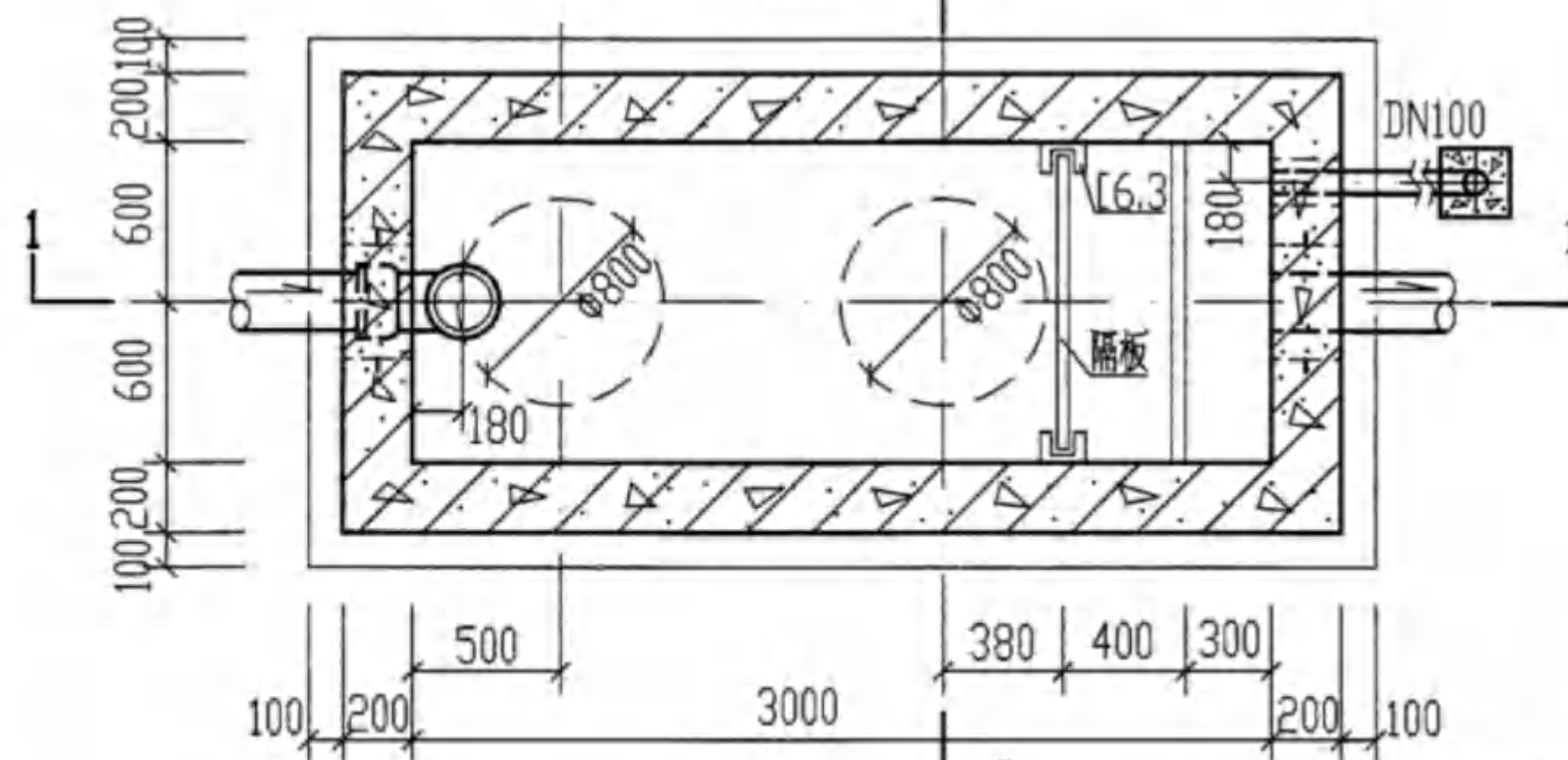
1型钢筋混凝土汽车洗车污水隔油沉淀池平、剖面图
