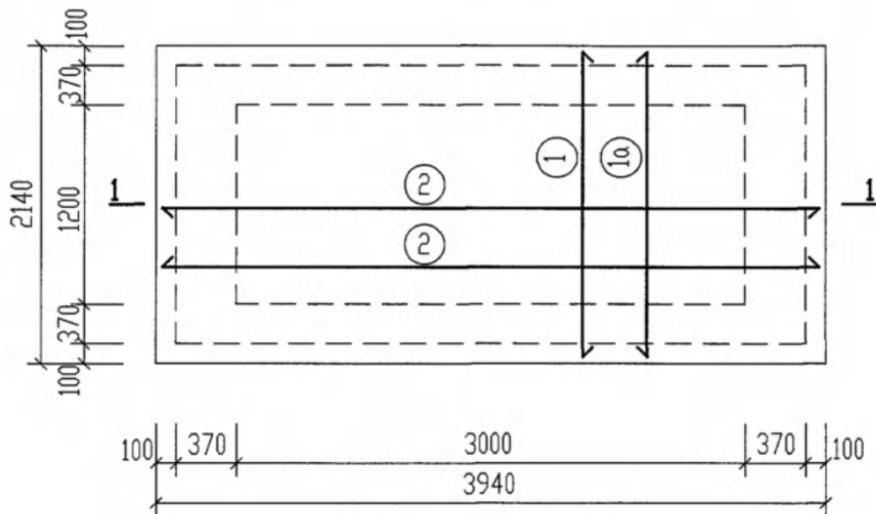
底板 DB-1 配筋图
