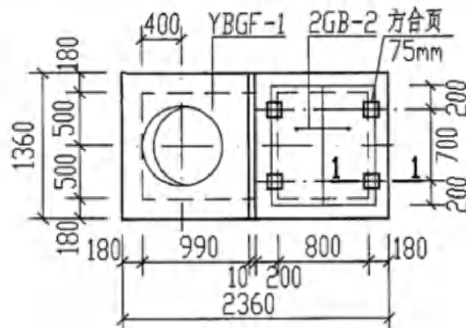
GG-2F. 2SF 盖板平面布置图
