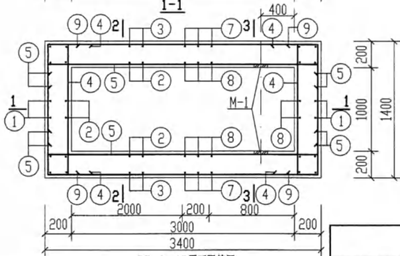
GG-4. 4S平面配筋图
