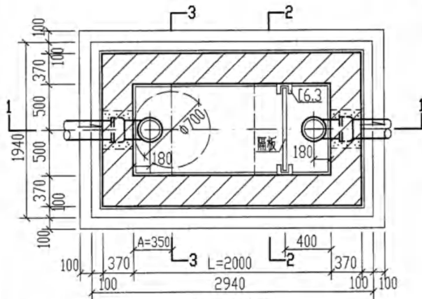
ZG-2F 平面图
