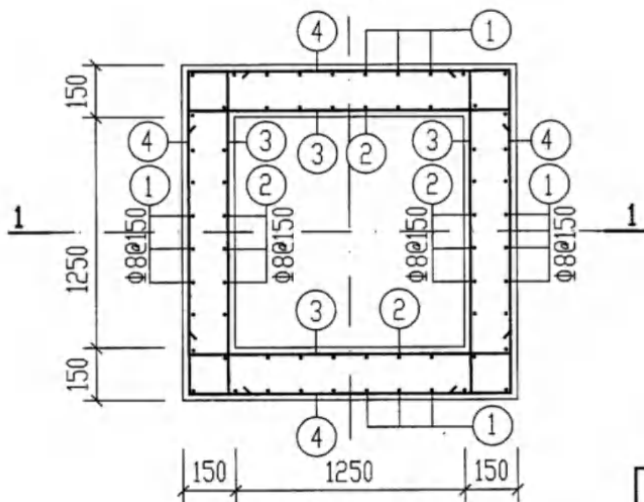
GJ-3 配筋图
