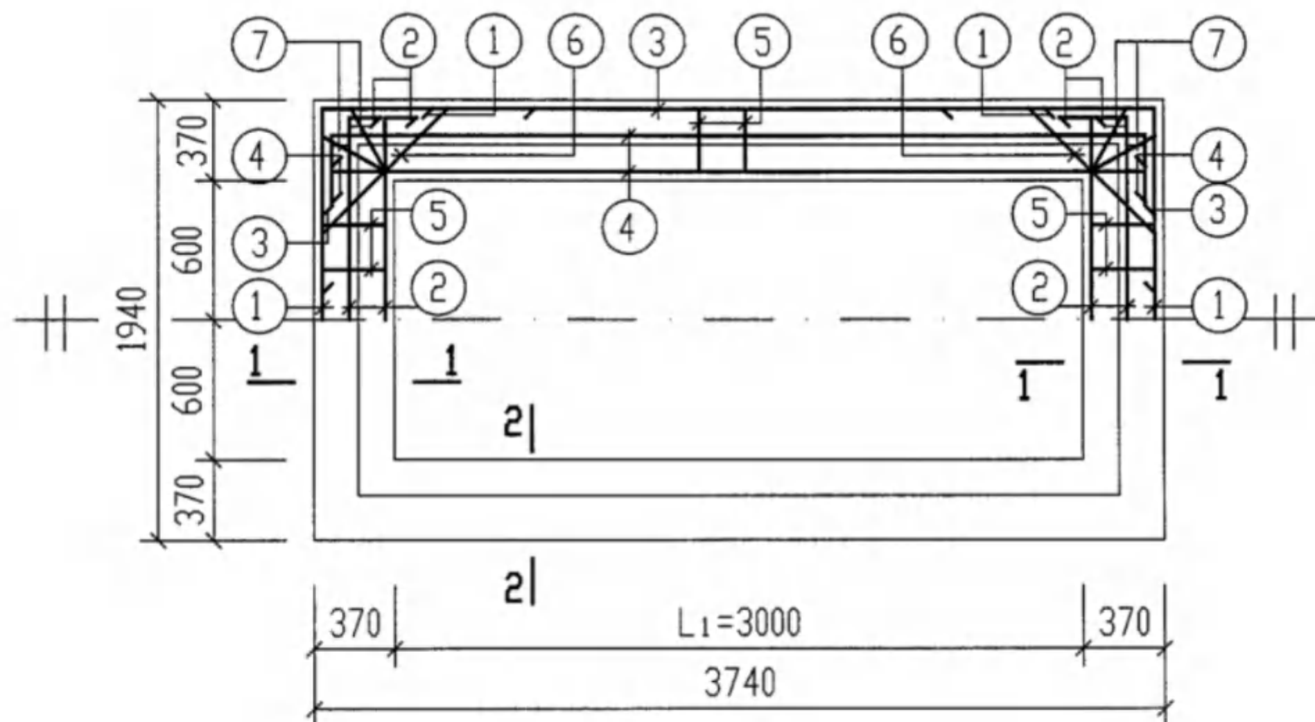
顶圈梁 DQL-1, 1a DQLF-1, 1a 配筋图
