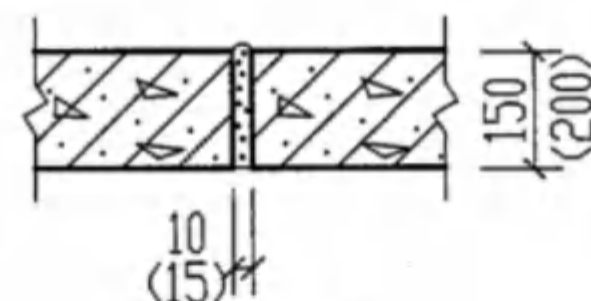
板缝示意图
