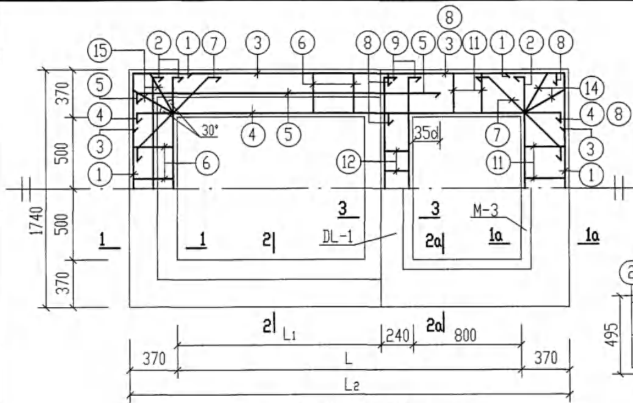
顶圈梁DQL-2~DQL-4配筋图
