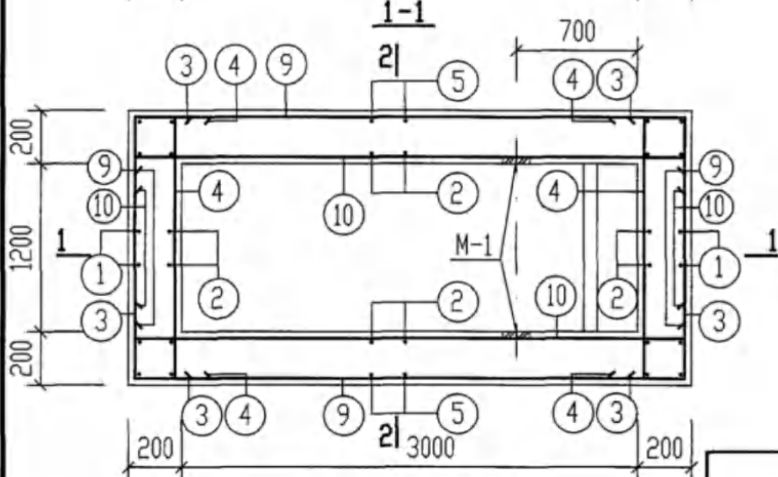
GC-1. 1S. 1Q. 1SQ平面配筋图
