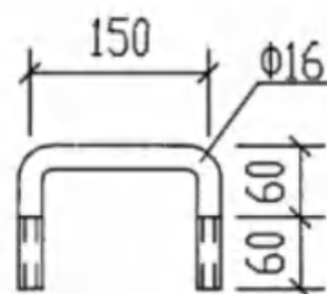
把手大样图
