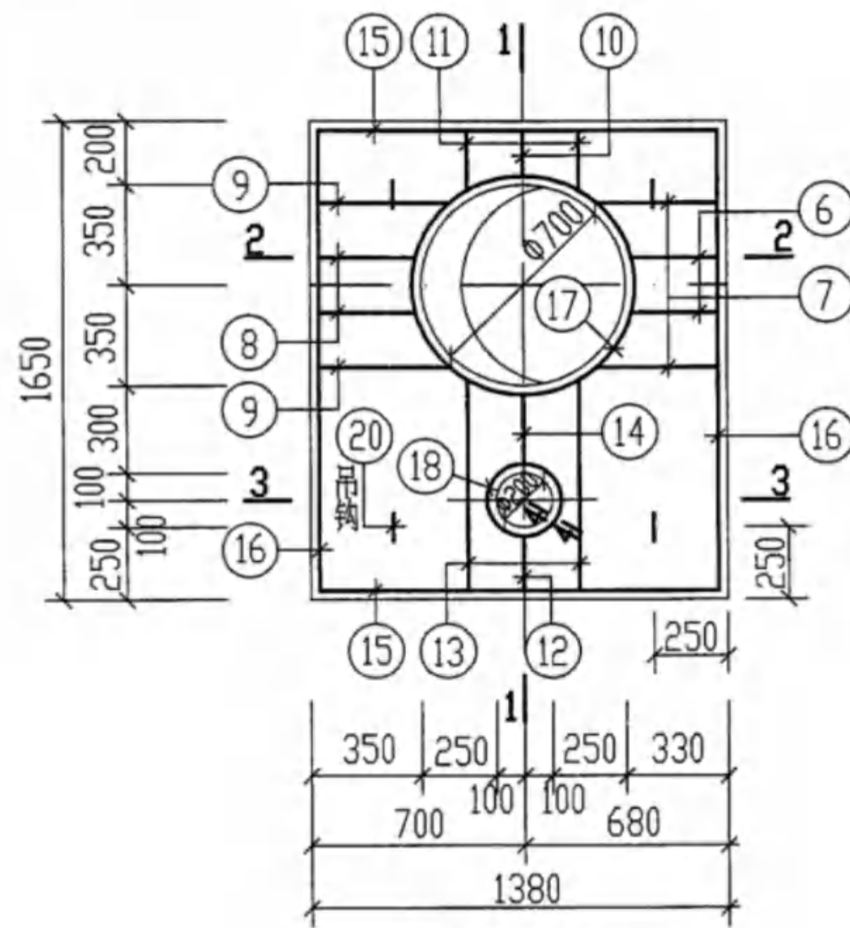
DGB-1. 4 上层钢筋
