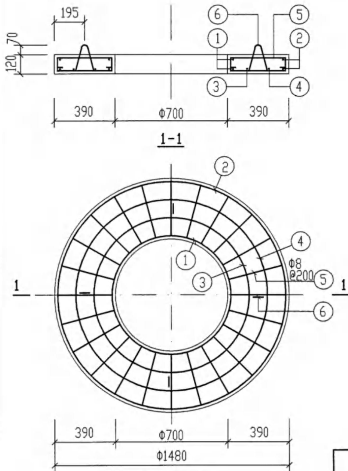
井圈(二)配筋图
