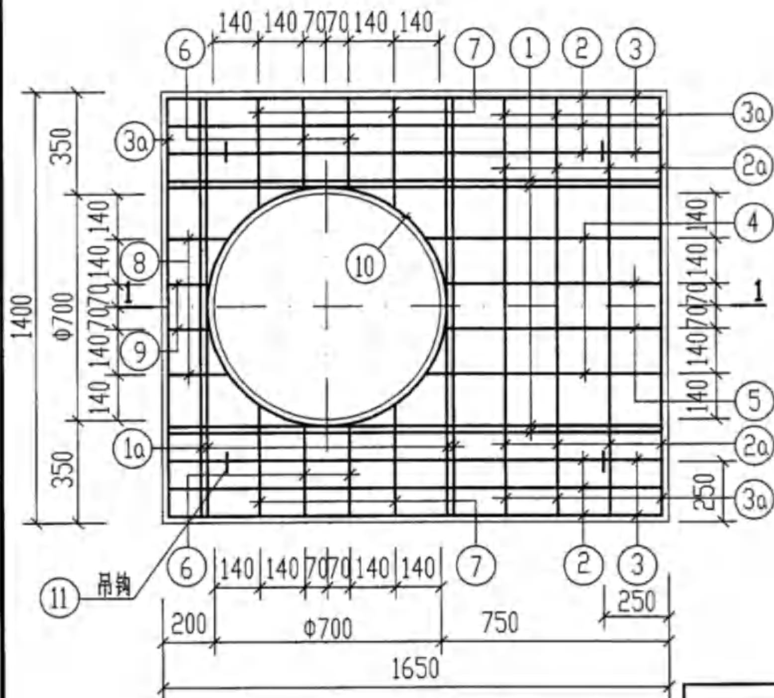
井圈(十一)配筋图
