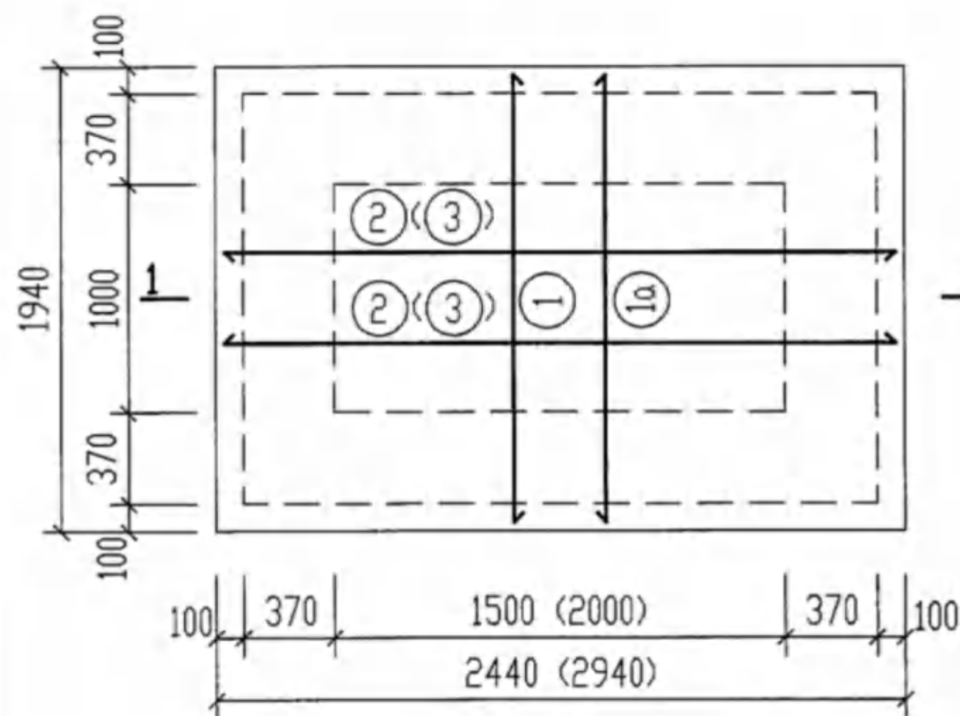
底板 DBF-1 (DBF-2) 配筋图
