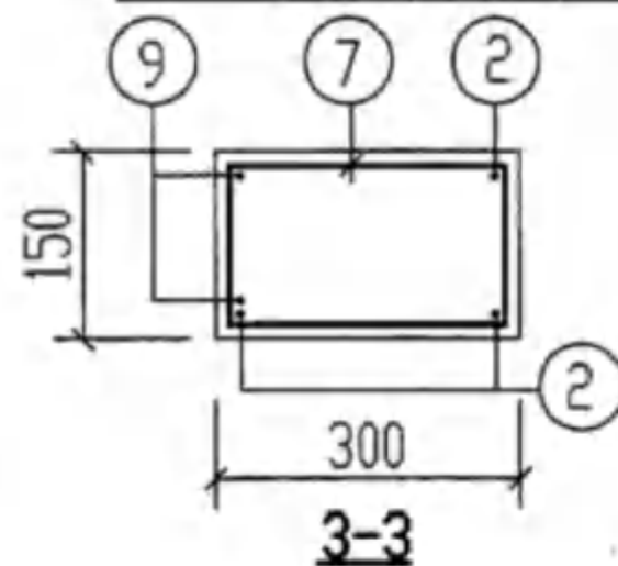
YBG-2, YBGF-2 配筋图
