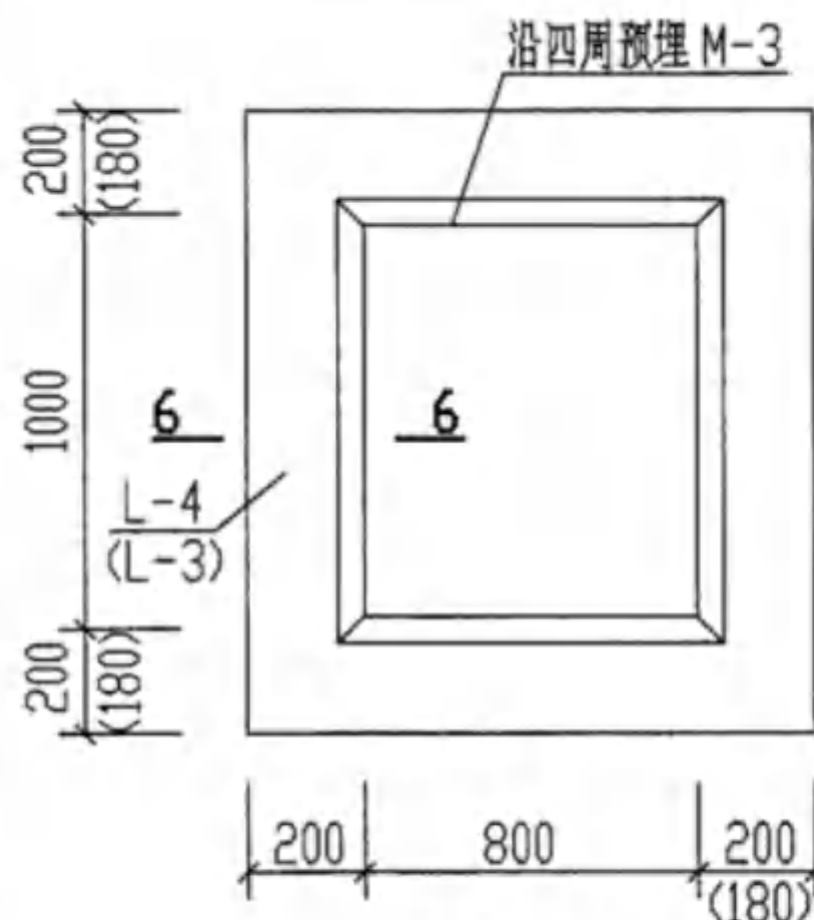
预埋件M-3平面图
