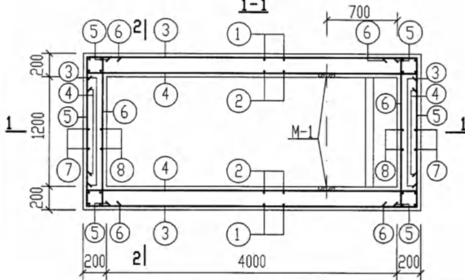
GC-2, 2S, 2Q, 2SQ平面配筋图
