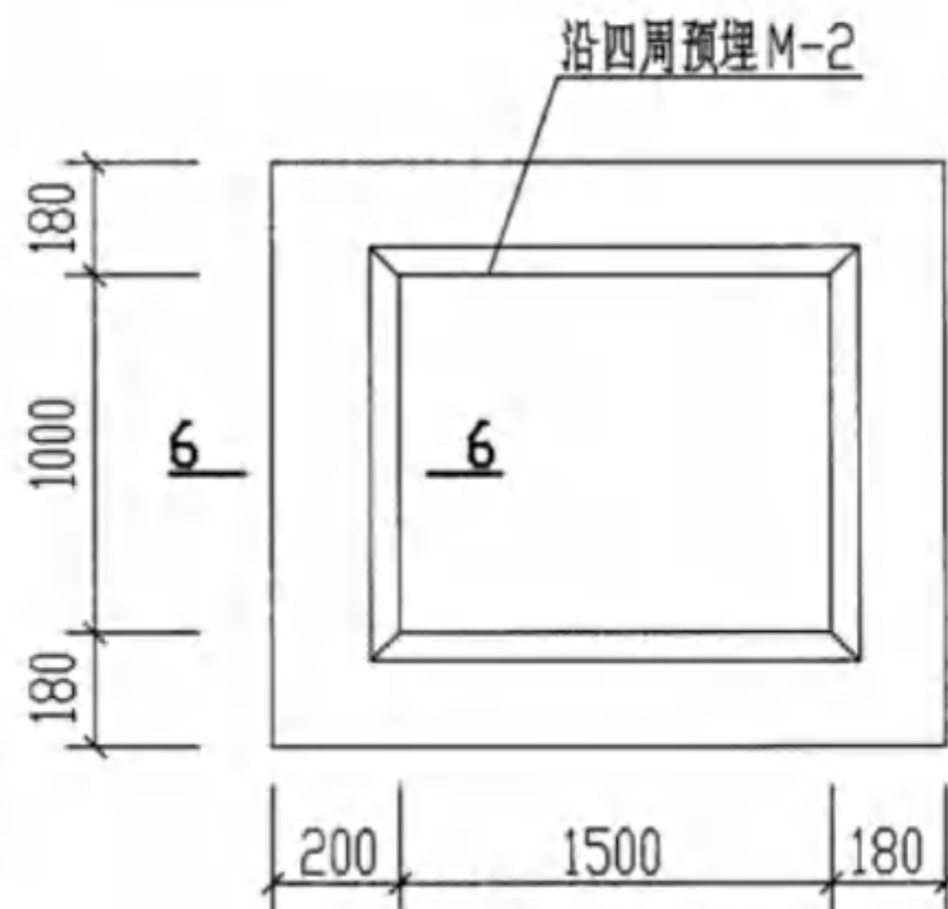
预埋件M-2平面图 (仅用于GG-1, 1S)
