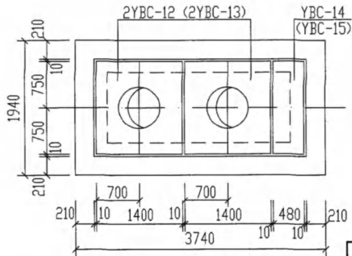
ZC-1. (ZC-1Q) 盖板平面布置图
