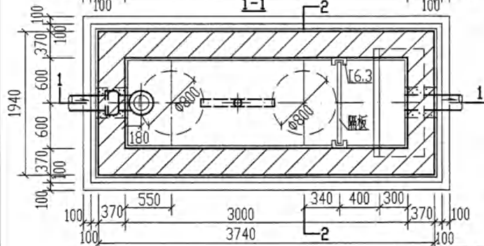
ZC-1F (ZC-1QF)平面图
