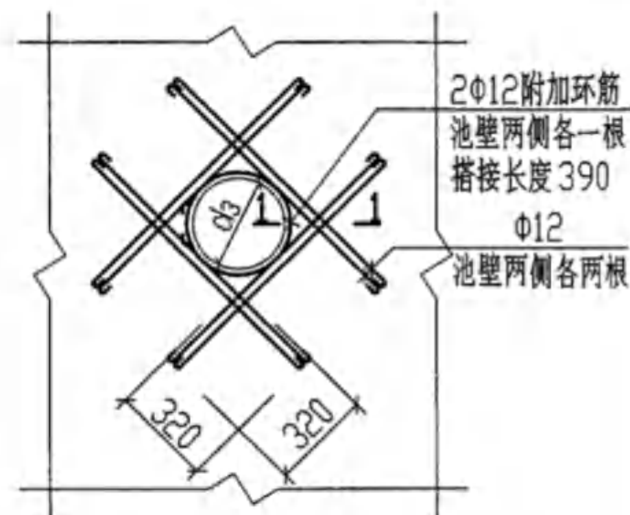
300 ≤ d 3 ≤ 1000 洞口加强大样图 (钢筋混凝土池壁)
