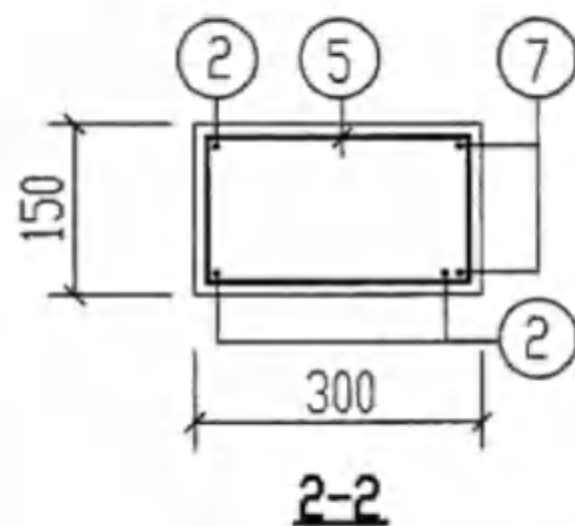
YBG-4. YBGF-4 配筋图 (无覆土和有覆土)
