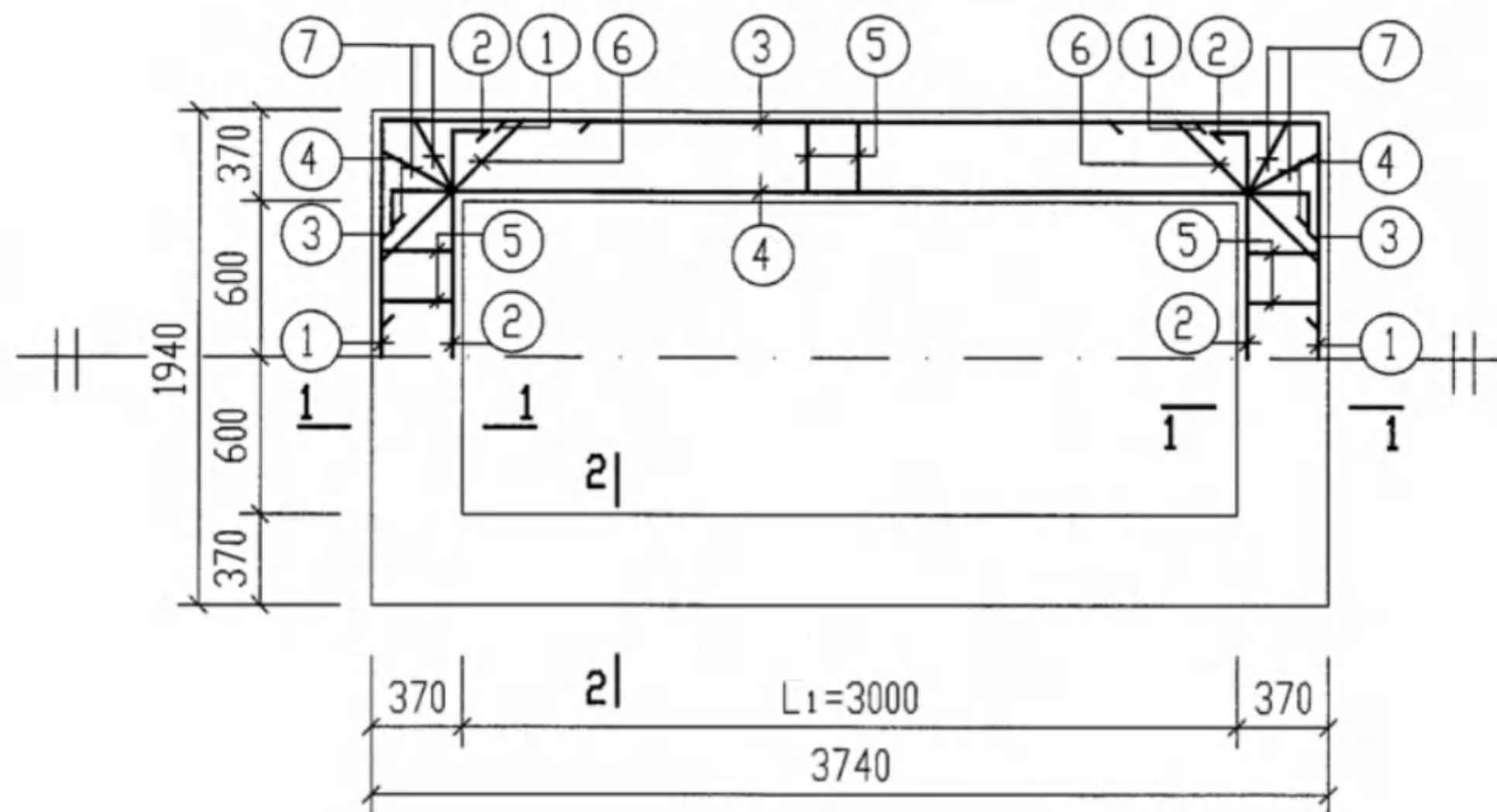
中圈梁ZQL-1. 1a ZQLF-1. 1a配筋图
