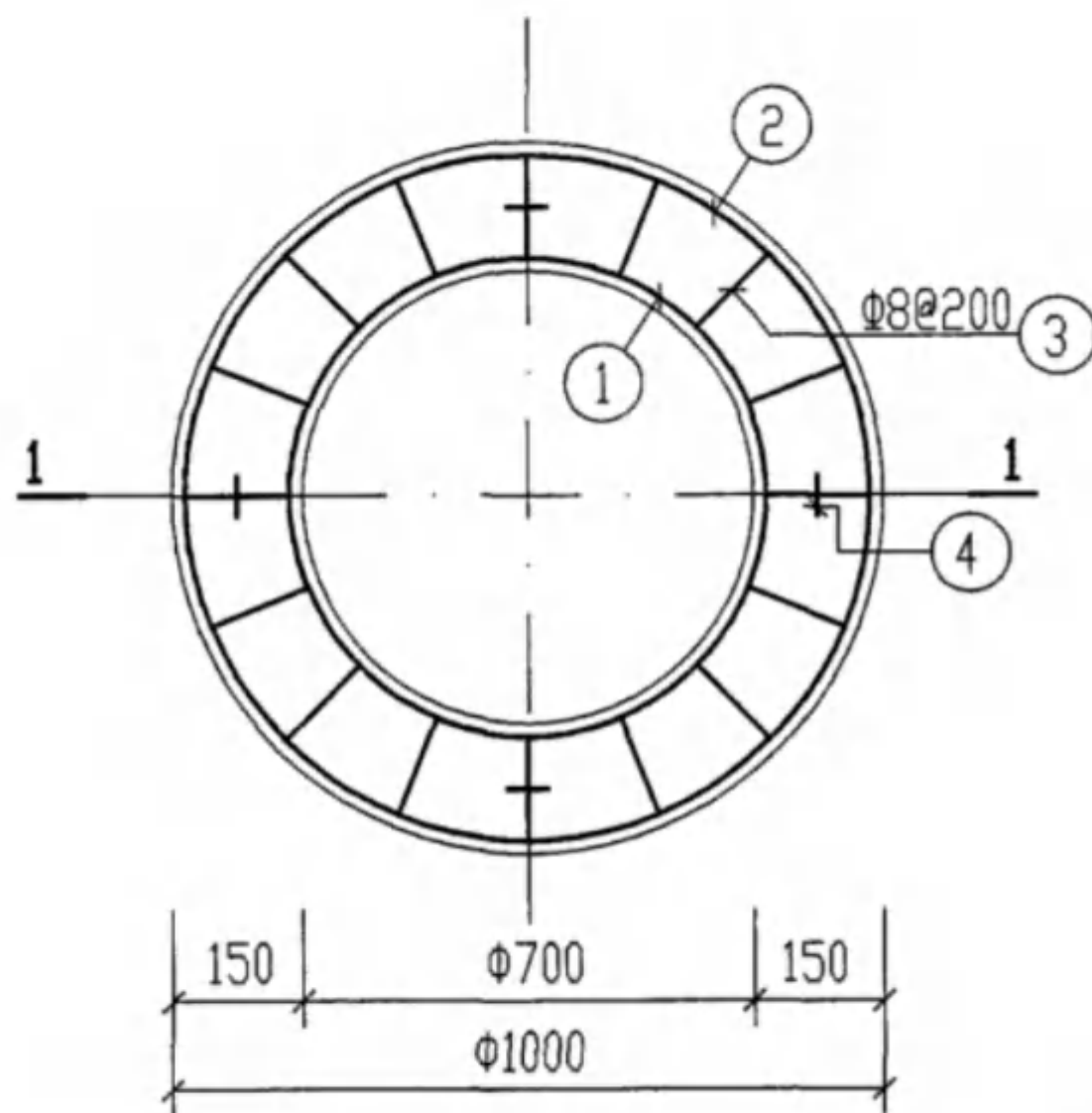
井圈(三)配筋图
