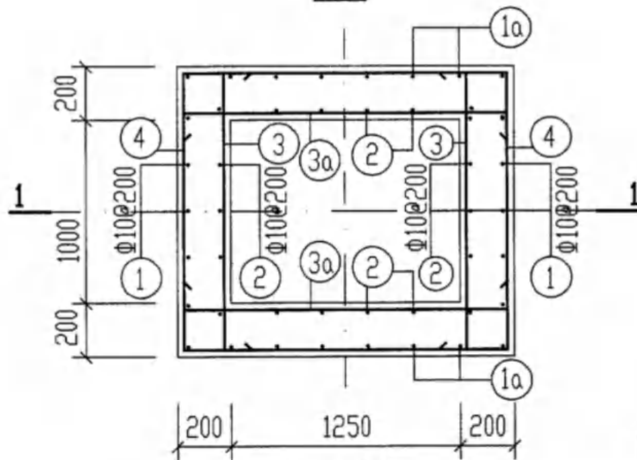
GS-2配筋图
