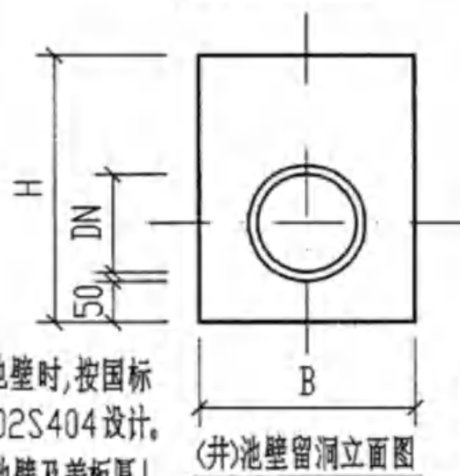
管道穿砖壁预留洞
