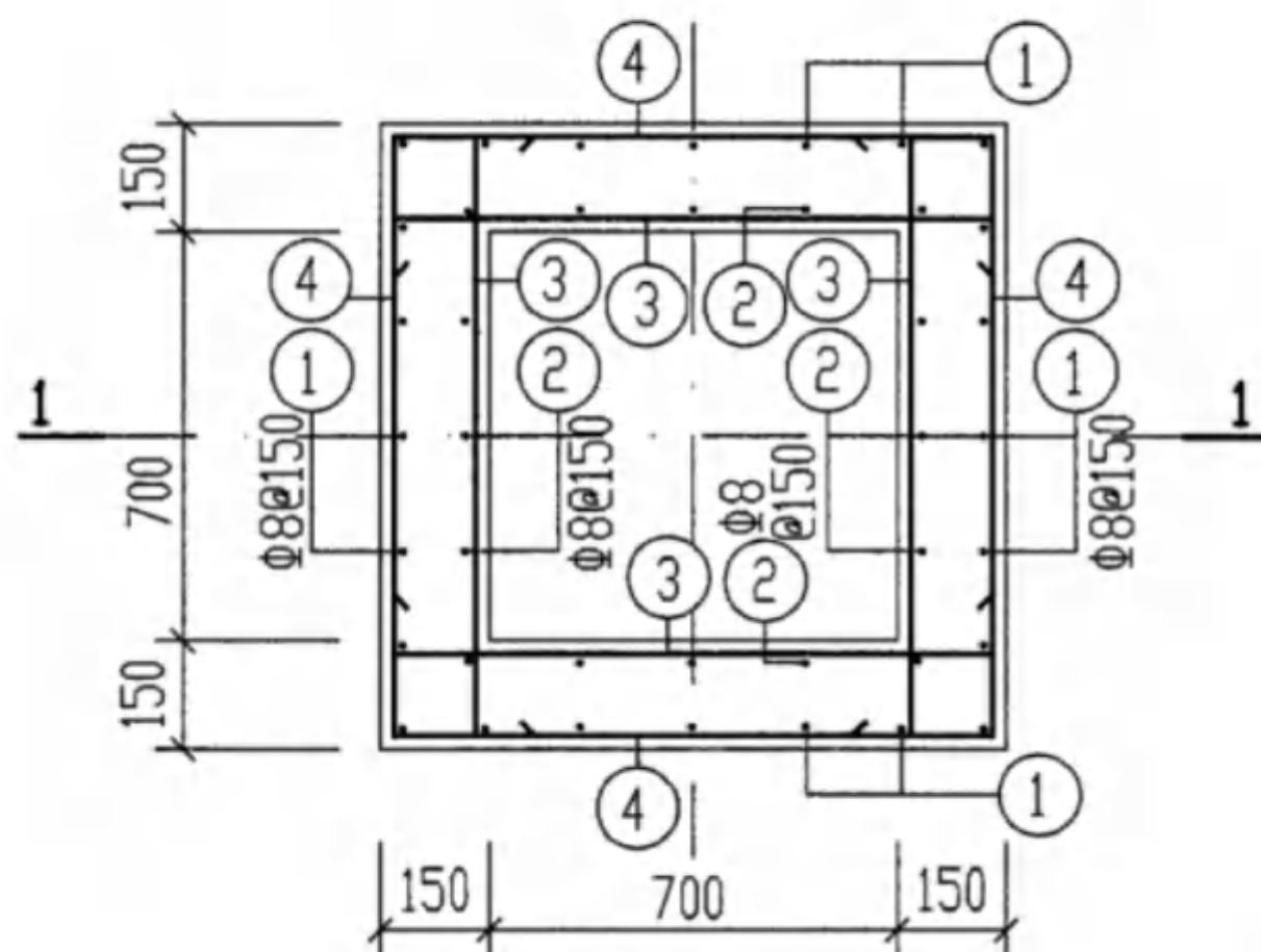
GJ-1配筋图
