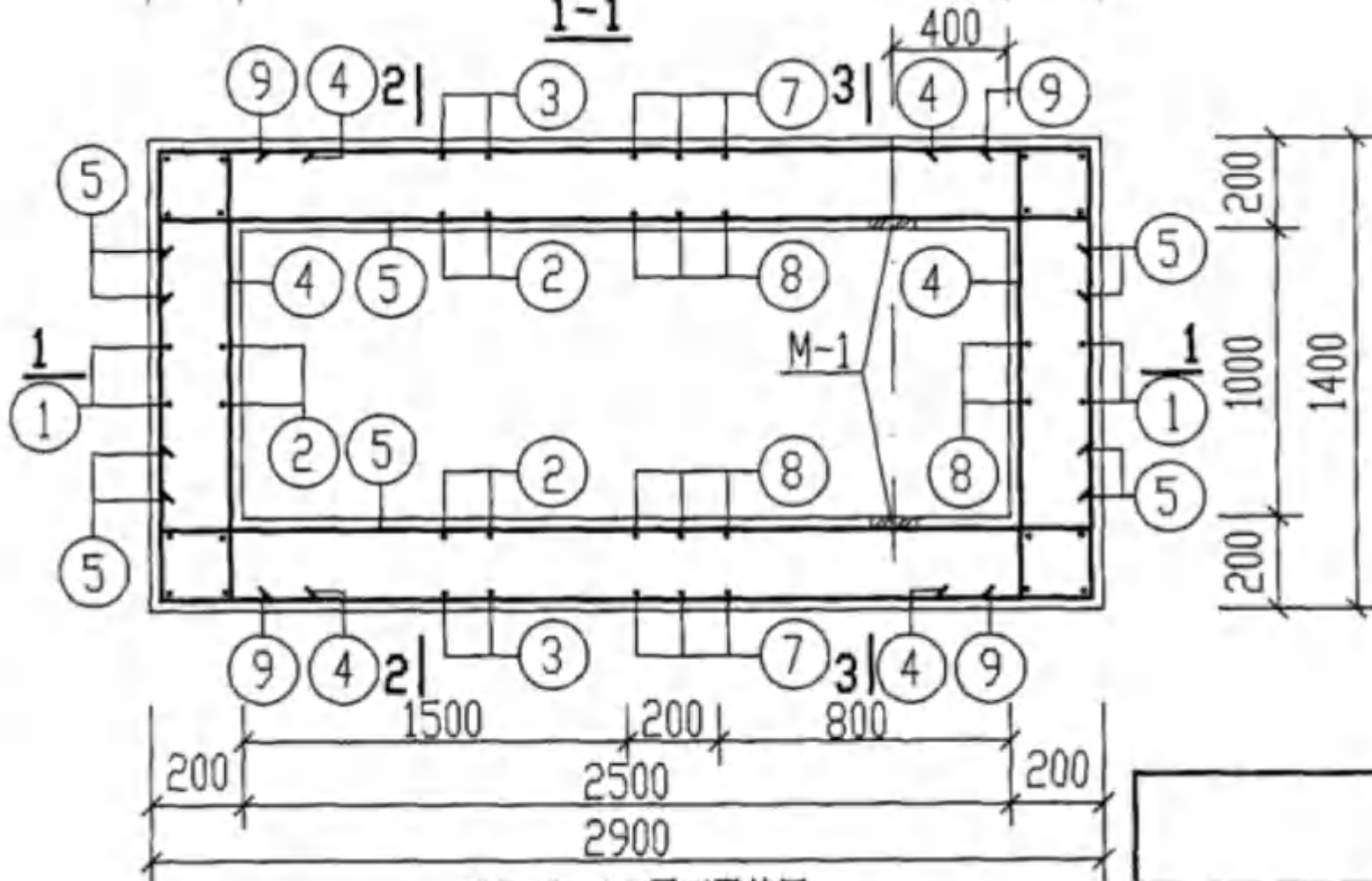
GG-3. 3S平面配筋图
