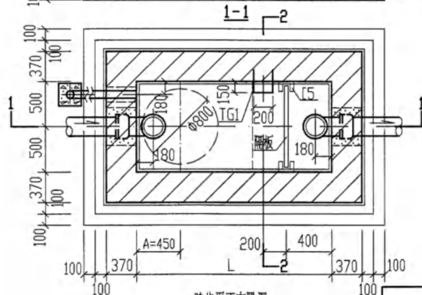
踏步平面布置图
