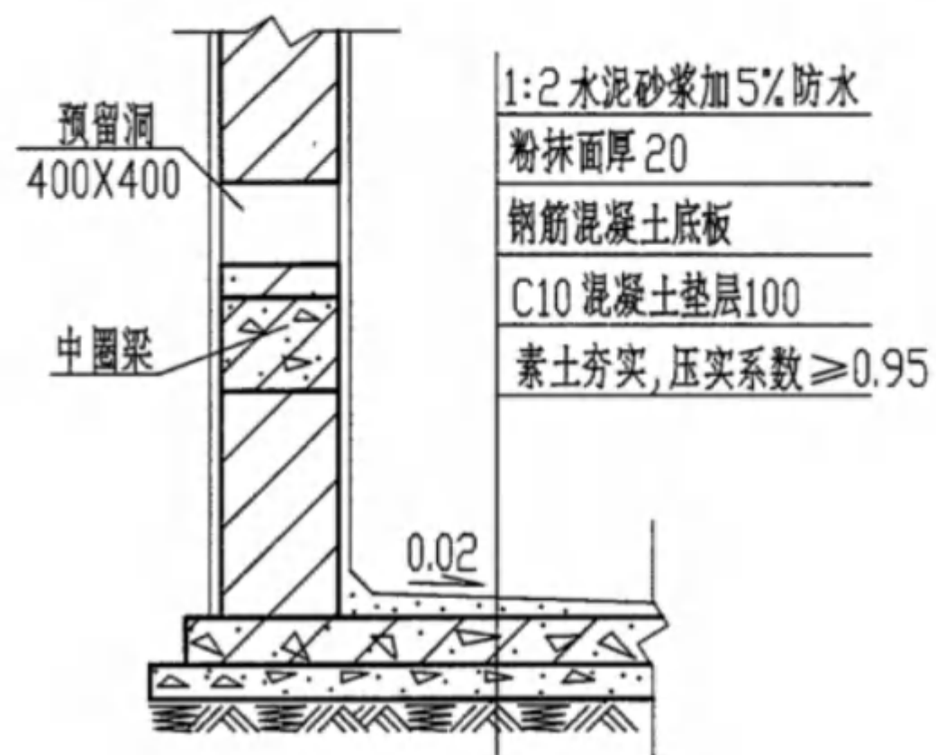
池底做法大样图 1-1 (用于无地下水)
