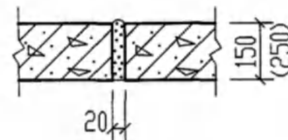
板缝示意图
