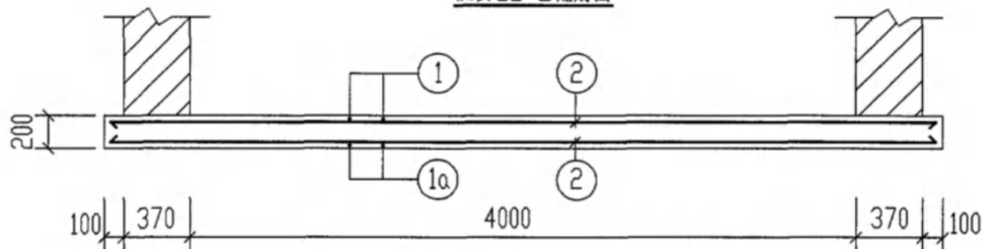
底板 DB-2 配筋图
