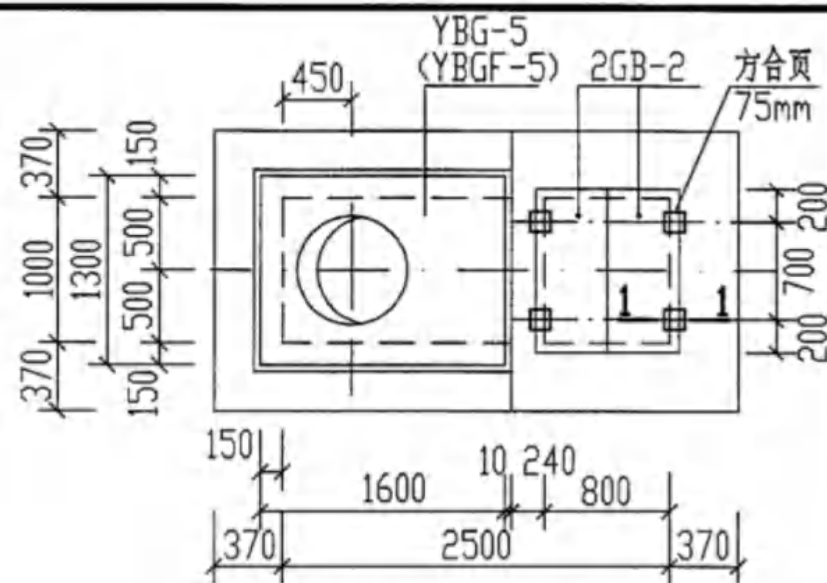
ZG-3. (ZG-3F) 盖板平面布置图
