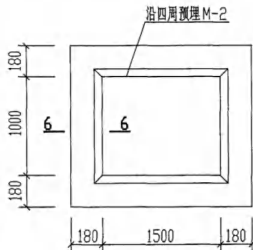
预埋件M-2平面图 (仅用于GG-1F, 1SF)
