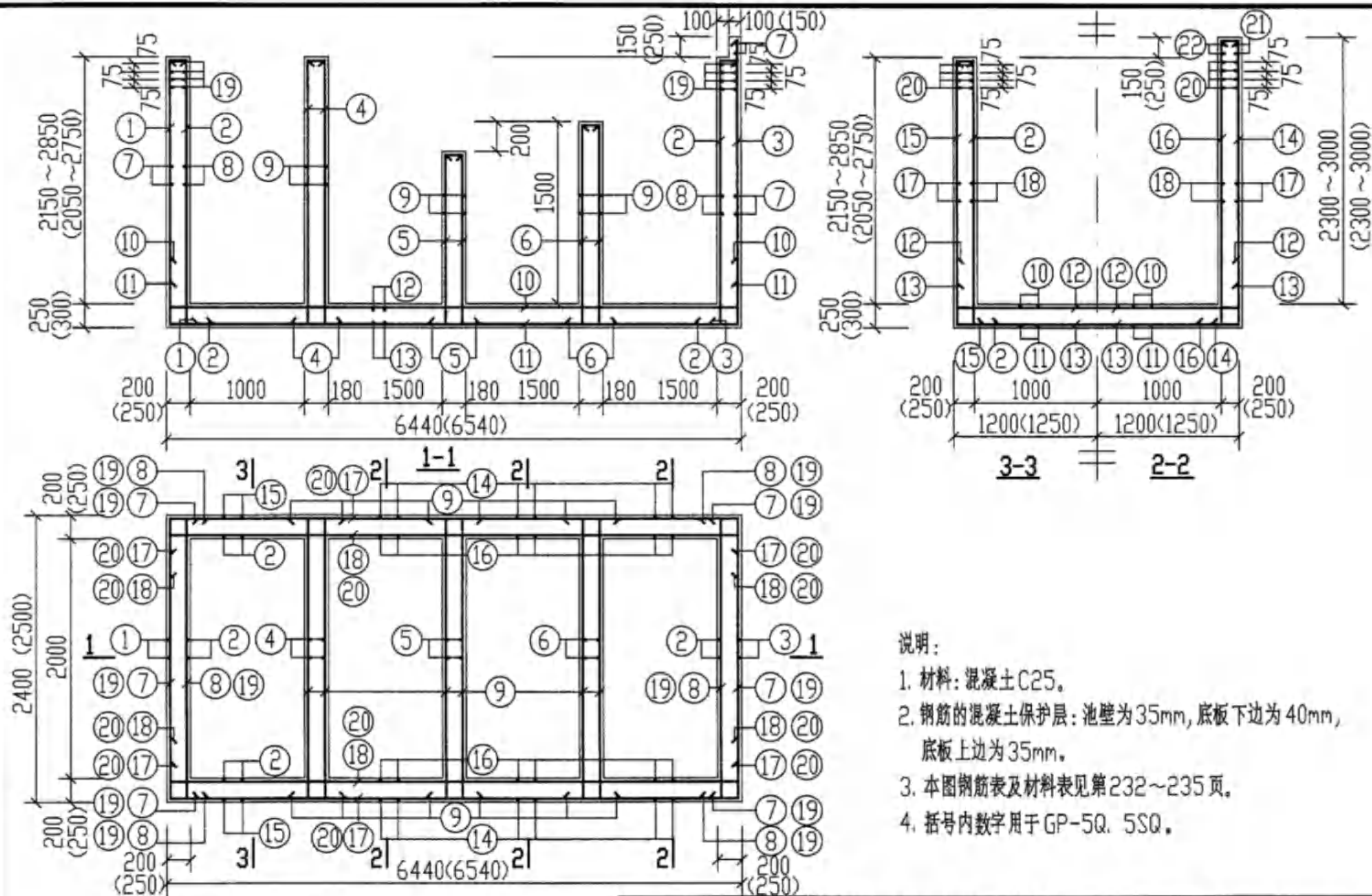
GP-5, 5S, 5Q, 5SQ配筋图 (无地下水和有地下水 顶面不过和可过汽车)
