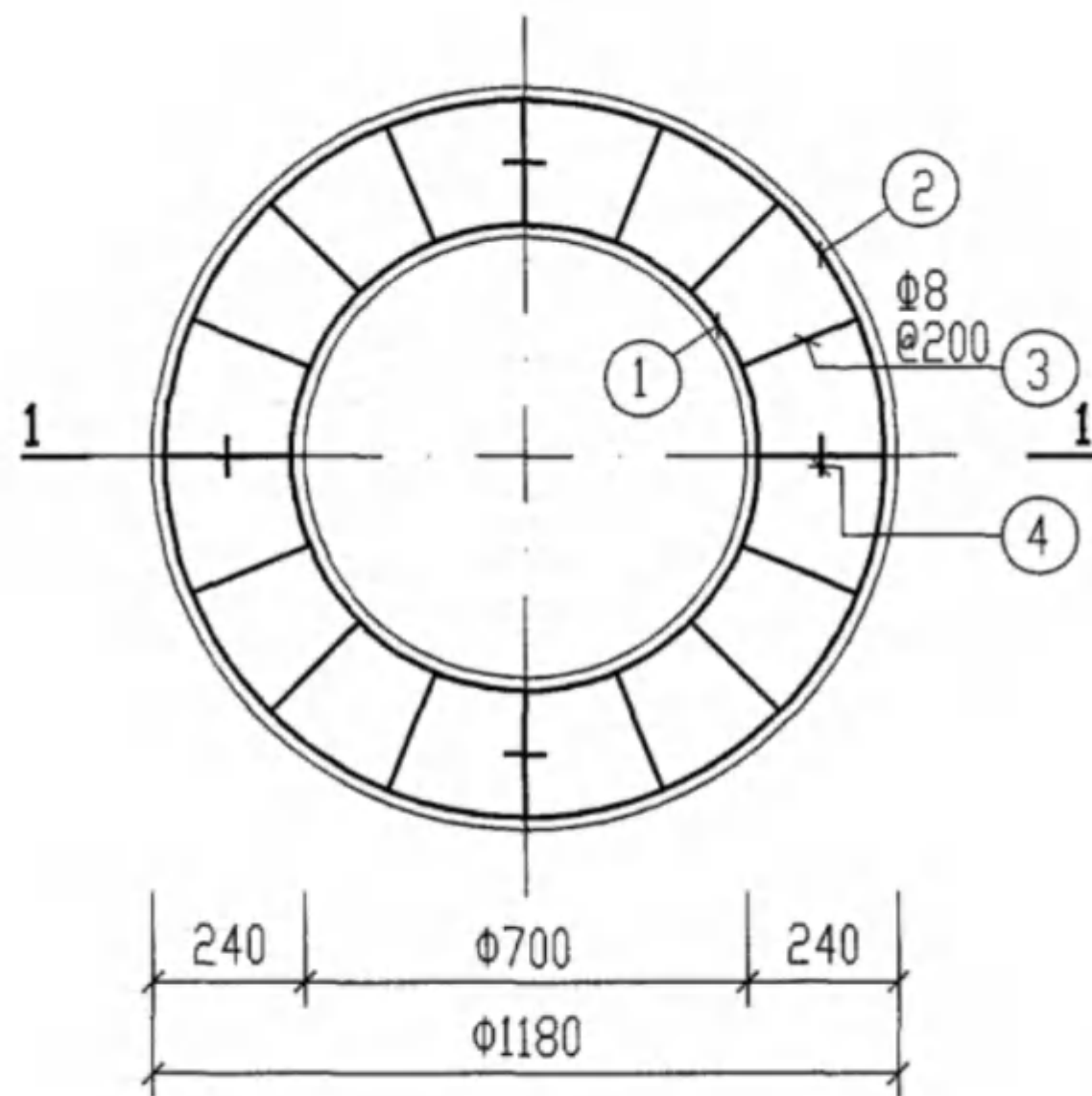
井圈(一)配筋图
