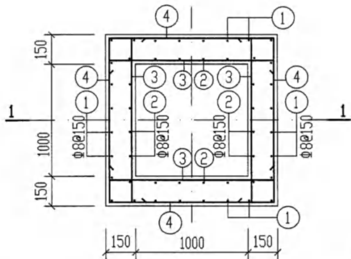
GJ-2配筋图
