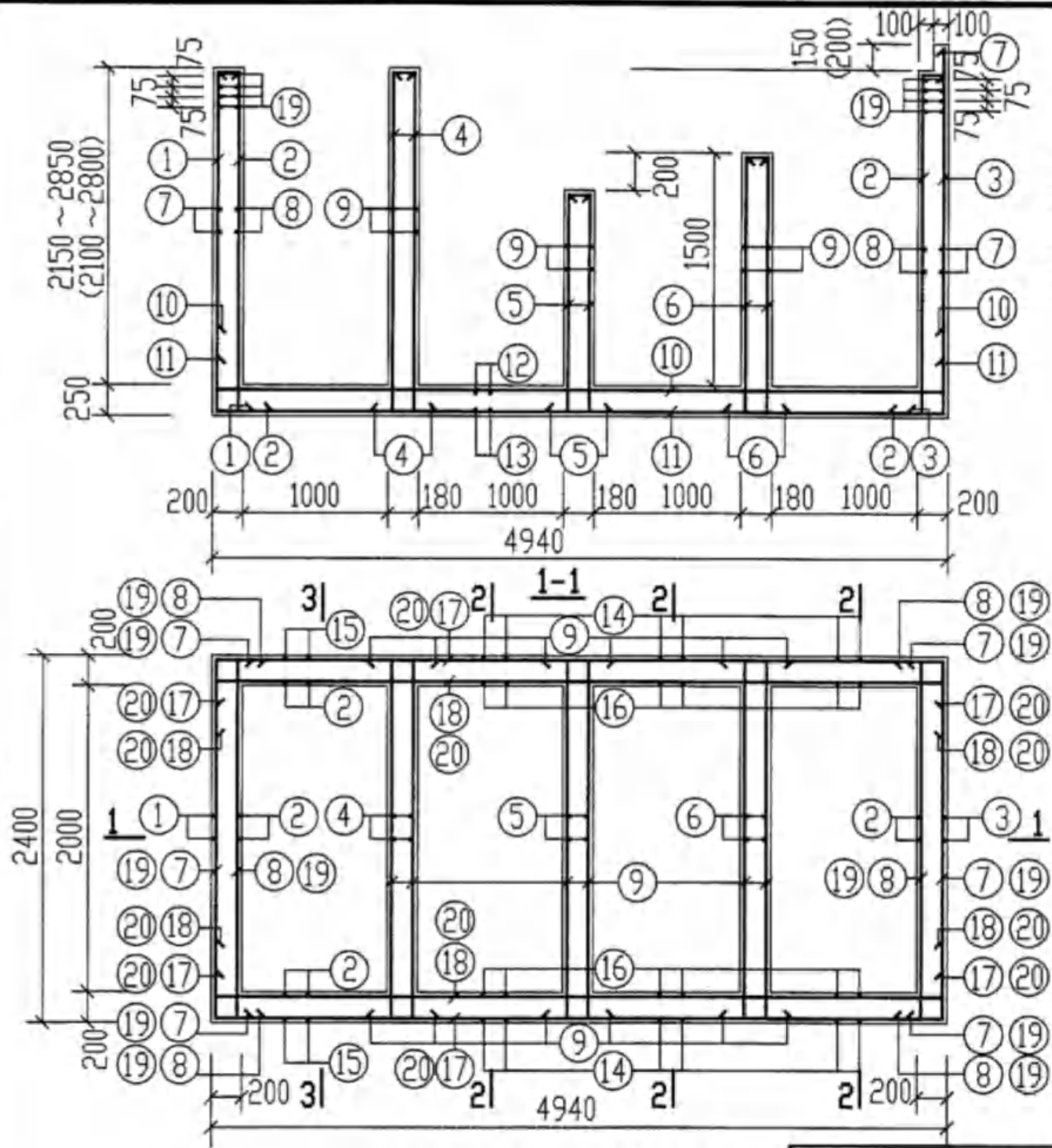
GP-4. 4S. 4Q. 4SQ 平面配筋图
