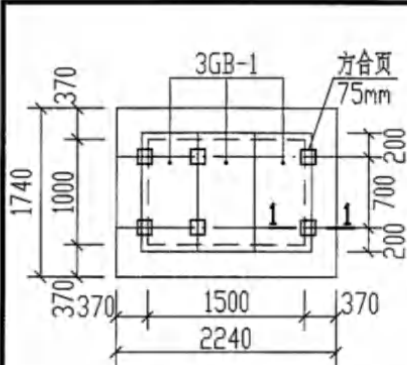
ZG-1. ZG-1F 盖板平面布置图
