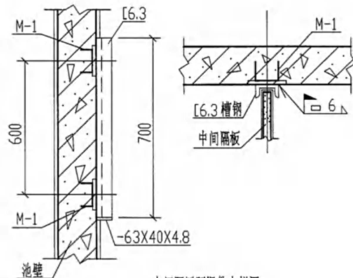
中间隔板预埋件大样图
