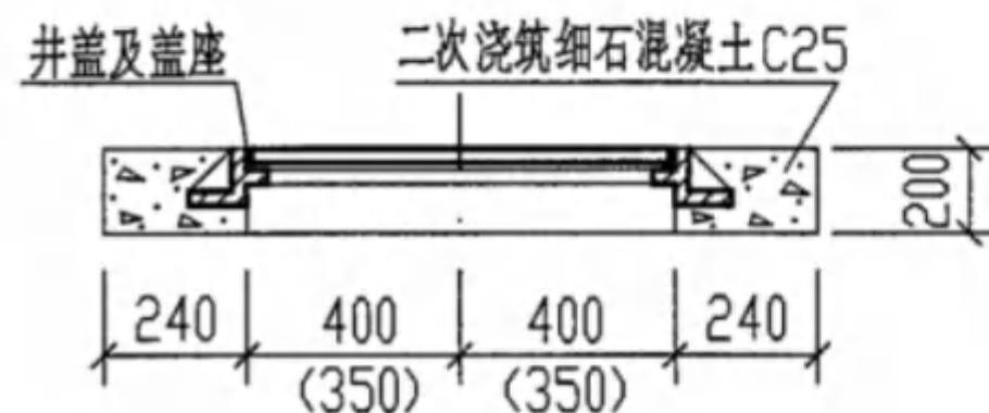
井盖及盖座安装图
