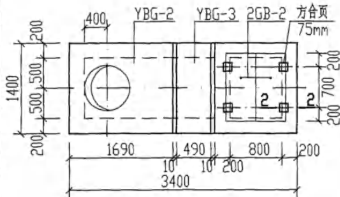
GG-4. 4S 盖板平面布置图
