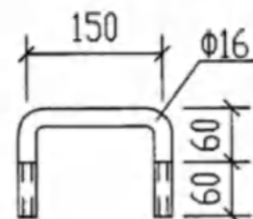
把手大样图
