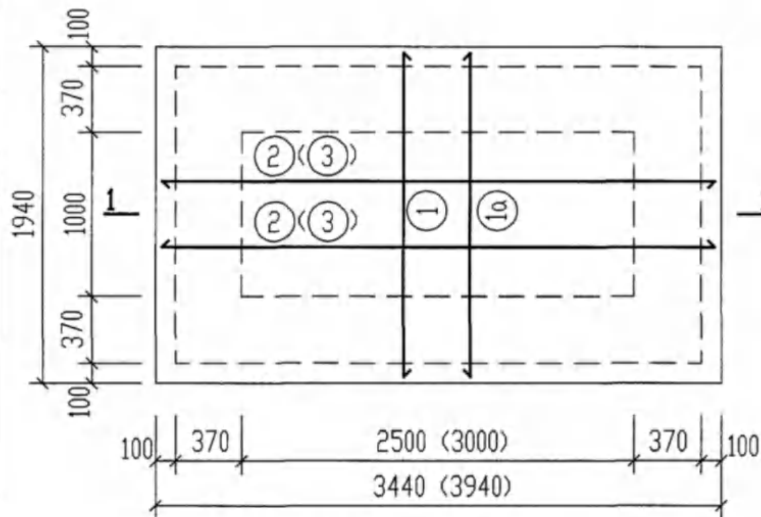
底板DB-3 (DB-4)配筋图
