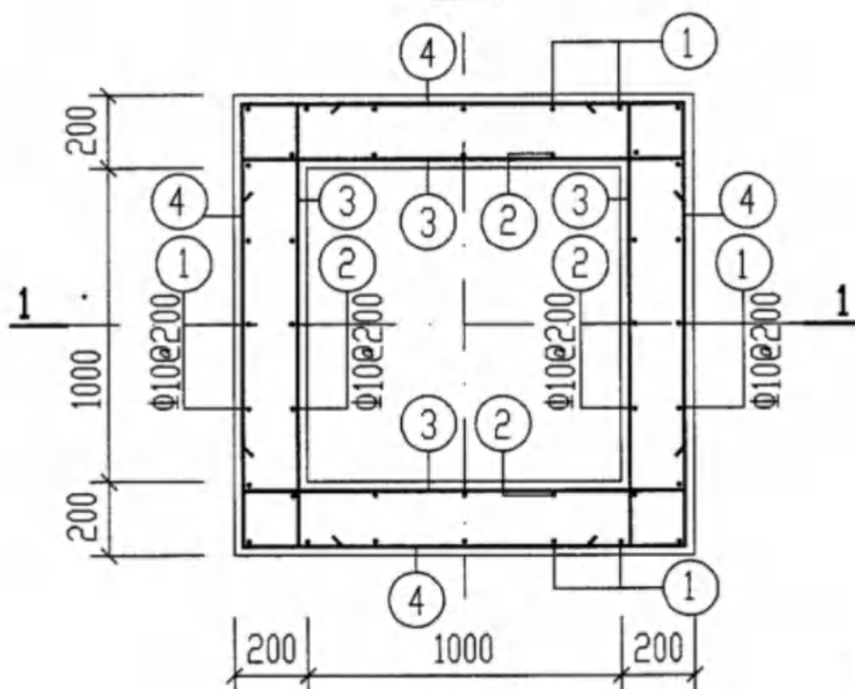
GS-1 配筋图
