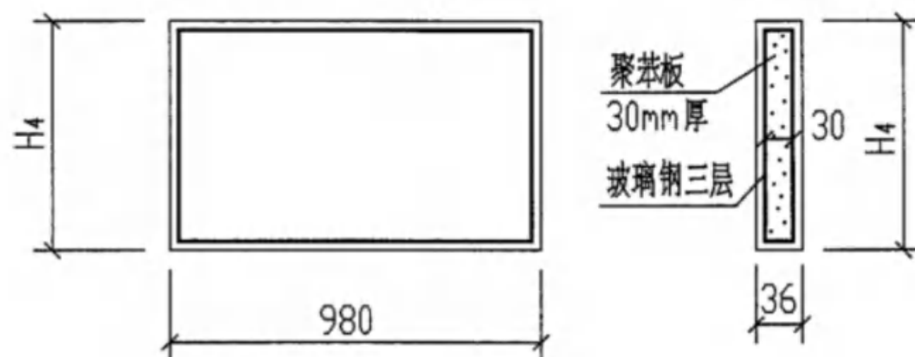
中间隔板大样图
