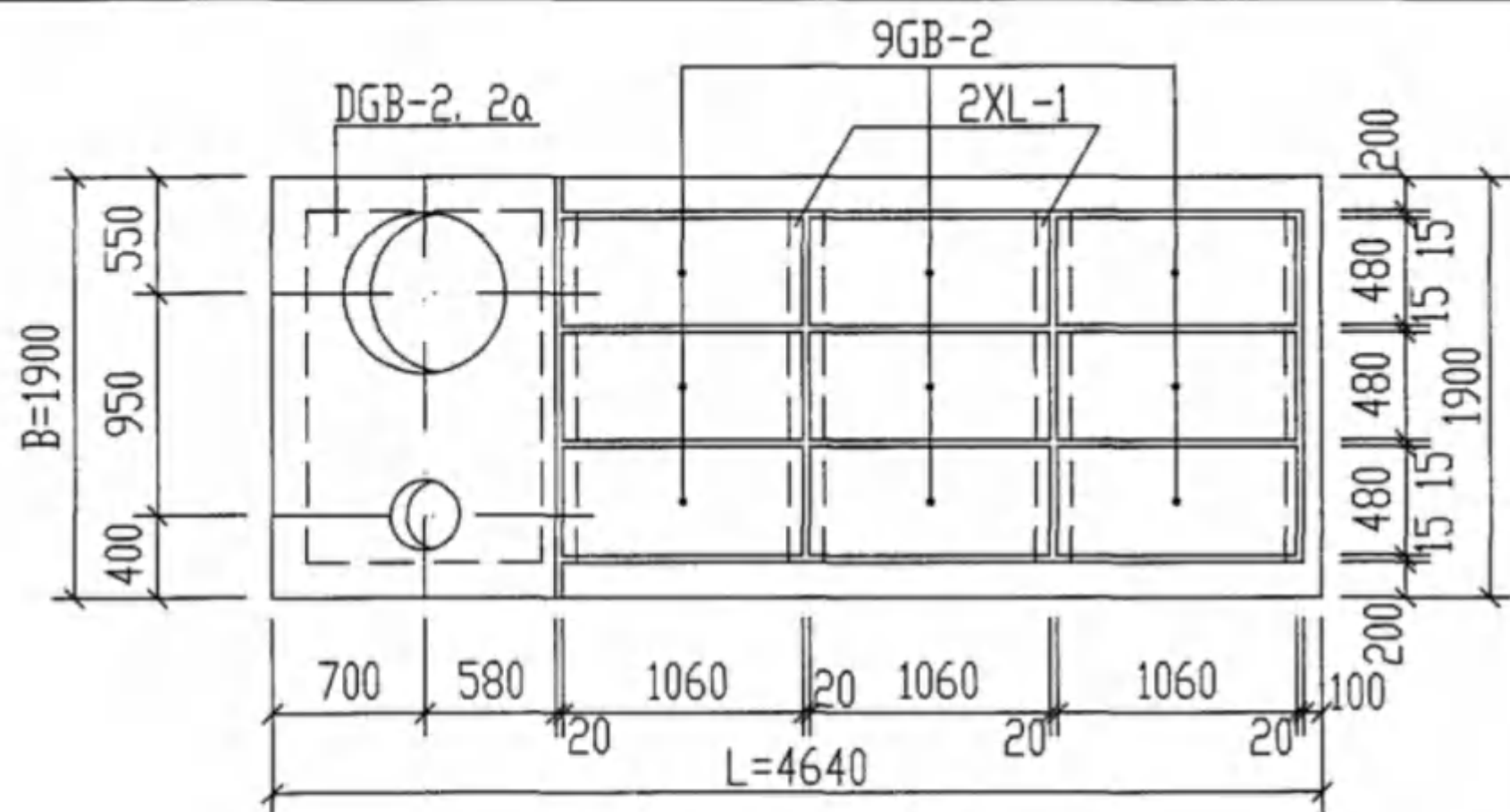
GP-3. 3S池盖板平面布置图
