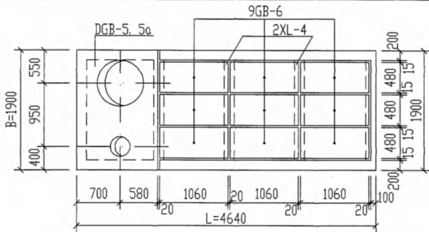
GP-3Q. 3SQ 池盖板平面布置图
