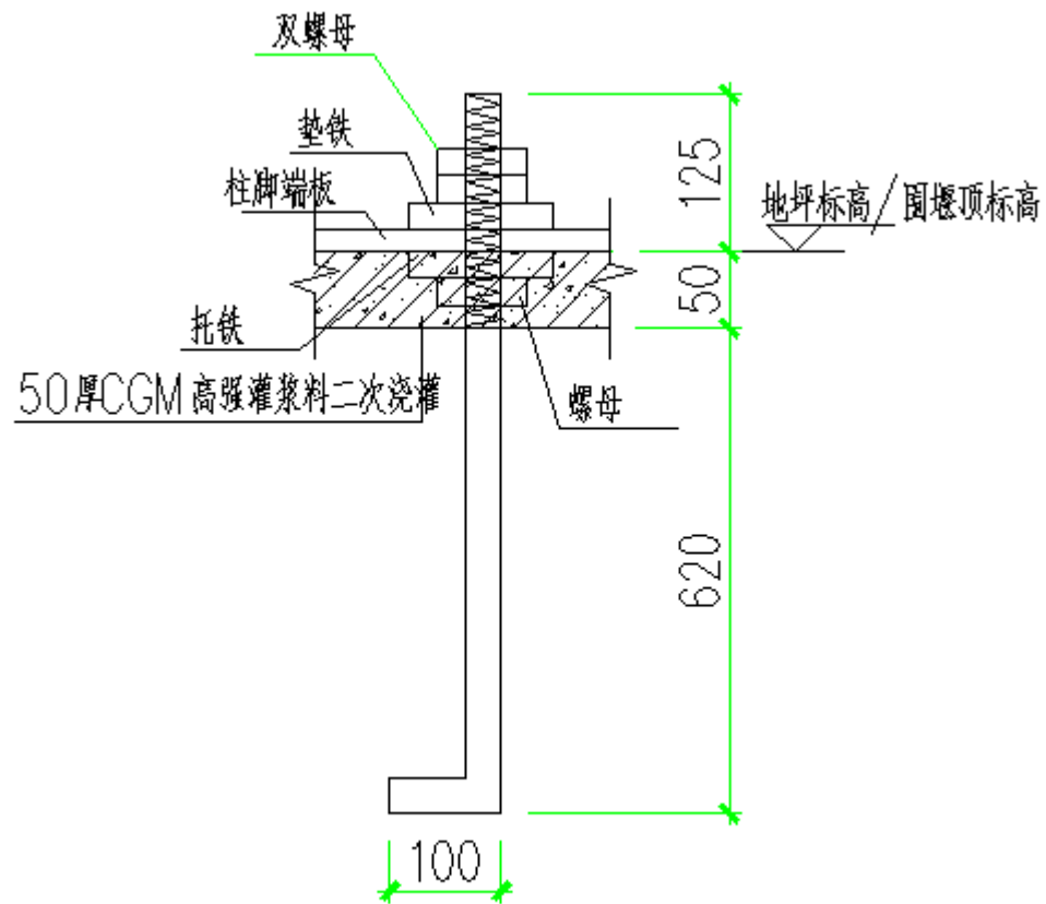
M24柱脚锚栓预埋简图
