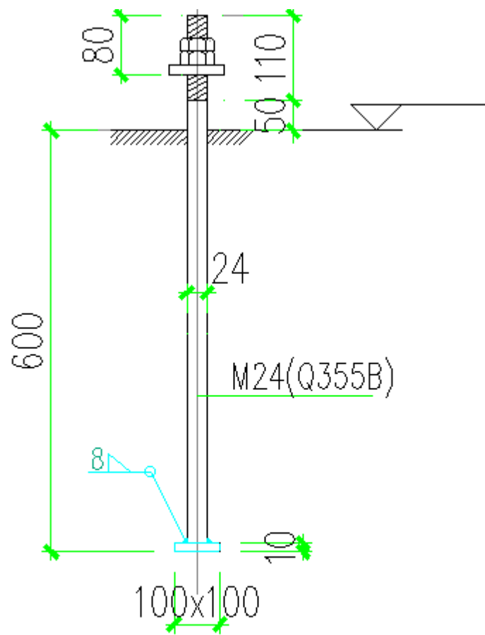
M24 锚栓示意图
